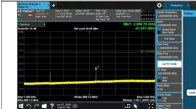
12-12-5MHz-10MHz-QPSK-QPSK-23038-23110-1RB#0-0RB#0-1 000~3000MHz-PASS
