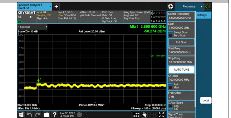
12-12-5MHz-5MHz-QPSK-QPSK-23071-23119-1RB#24-0RB#0-3 000~10000MHz-PASS
