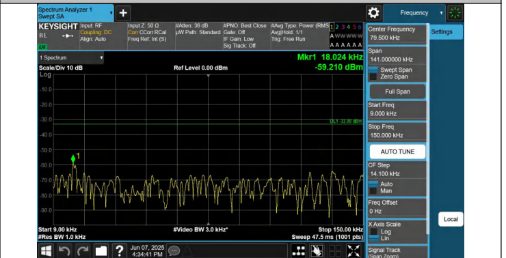
12-12-5MHz-5MHz-QPSK-QPSK-23071-23119-1RB#24-0RB#0-0. 009~0.15MHz-PASS
