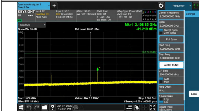
12-12-5MHz-5MHz-QPSK-QPSK-23071-23119-1RB#0-0RB#0-10 00~3000MHz-PASS
