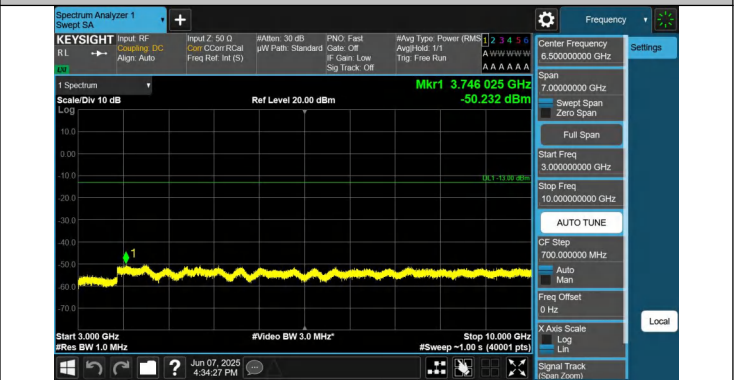
12-12-5MHz-5MHz-QPSK-QPSK-23071-23119-1RB#0-0RB#0-30 00~10000MHz-PASS
