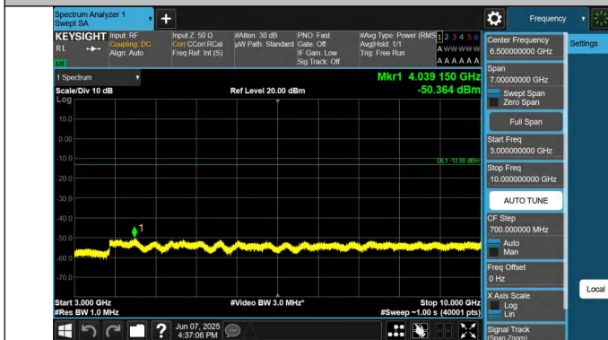
12-12-5MHz-5MHz-QPSK-QPSK-23107-23155-1RB#24-0RB#0-3 000~10000MHz-PASS
