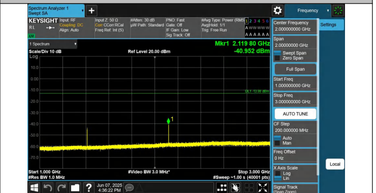
12-12-5MHz-5MHz-QPSK-QPSK-23107-23155-1RB#0-0RB#0-10 00~3000MHz-PASS
