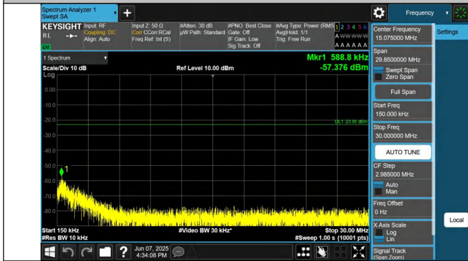
12-12-5MHz-5MHz-QPSK-QPSK-23071-23119-1RB#0-0RB#0-0. 15~30MHz-PASS
