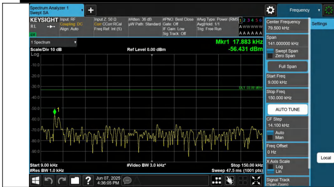
12-12-5MHz-5MHz-QPSK-QPSK-23107-23155-1RB#0-0RB#0-0. 009~0.15MHz-PASS
