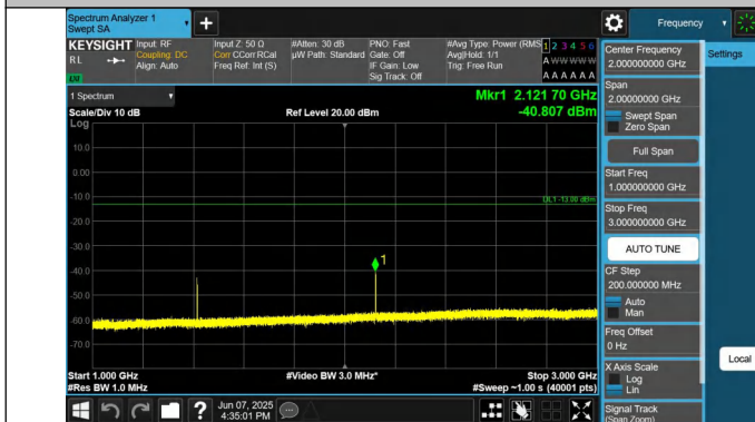
12-12-5MHz-5MHz-QPSK-QPSK-23071-23119-1RB#24-0RB#0-1 000~3000MHz-PASS
