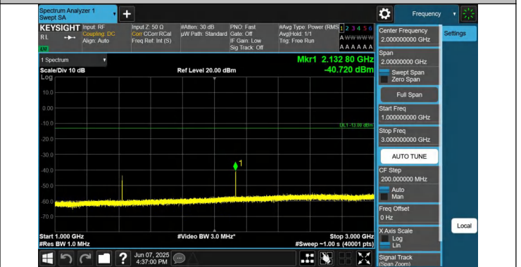
12-12-5MHz-5MHz-QPSK-QPSK-23107-23155-1RB#24-0RB#0-1 000~3000MHz-PASS
