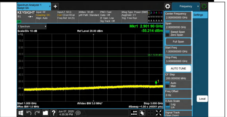
12-12-5MHz-5MHz-QPSK-QPSK-23071-23119-1RB#0-1RB#24-1 000~3000MHz-PASS
