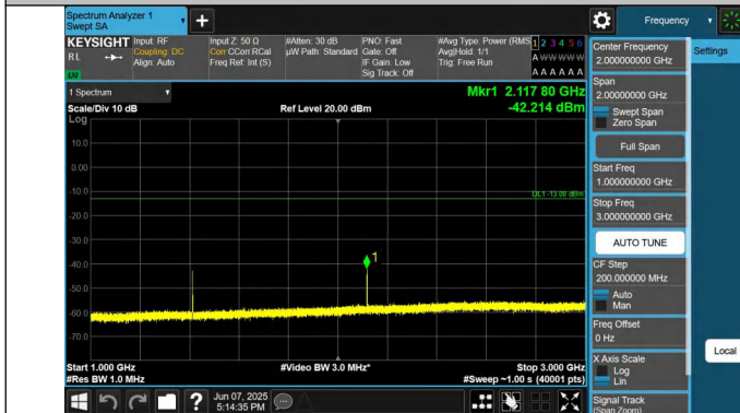
12-12-5MHz-10MHz-QPSK-QPSK-23058-23130-1RB#24-0RB#0- 1000~3000MHz-PASS
