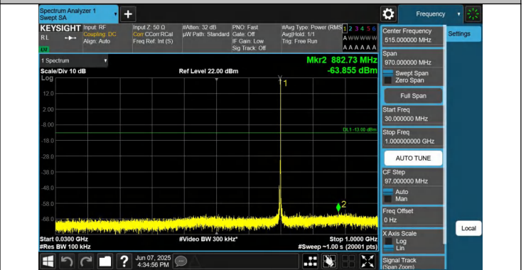
12-12-5MHz-5MHz-QPSK-QPSK-23071-23119-1RB#24-0RB#0-3 0~1000MHz-PASS
