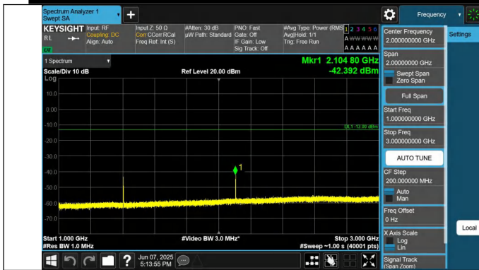
12-12-5MHz-10MHz-QPSK-QPSK-23058-23130-1RB#0-0RB#0-1 000~3000MHz-PASS
