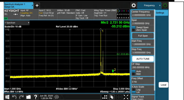
7-7-20MHz-20MHz-QPSK-QPSK-21001-21199-1RB#0-1RB#99-1 000~3000MHz-PASS
