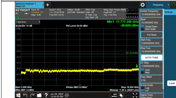
000~18000MHz-PASS
