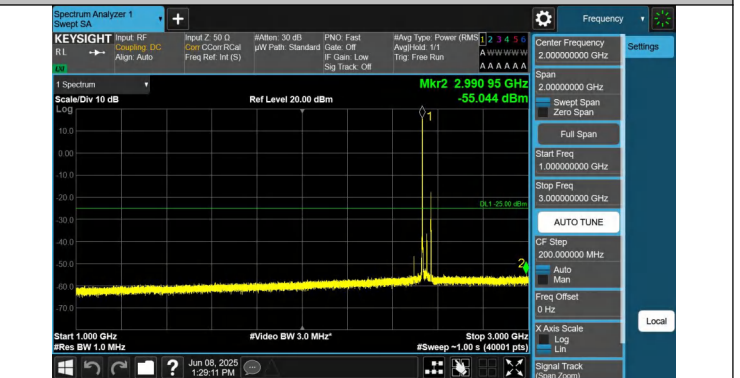
7-7-20MHz-20MHz-QPSK-QPSK-21152-21350-1RB#0-1RB#99-1 000~3000MHz-PASS
