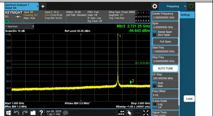
7-7-20MHz-20MHz-QPSK-QPSK-21001-21199-1RB#99-0RB#0-1 000~3000MHz-PASS
