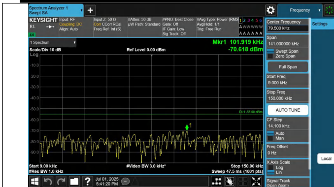
7-7-20MHz-20MHz-QPSK-QPSK-21001-21199-1RB#0-0RB#0-0. 009~0.15MHz-PASS
