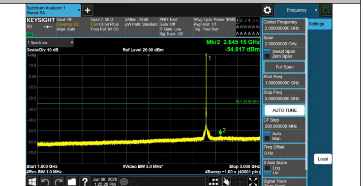
7-7-20MHz-20MHz-QPSK-QPSK-21001-21199-1RB#0-0RB#0-10 00~3000MHz-PASS
