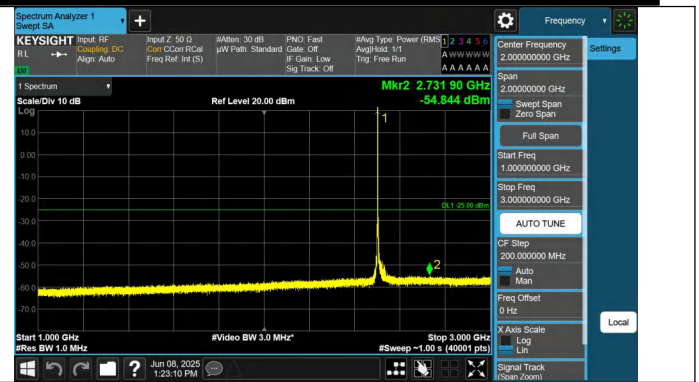
7-7-20MHz-20MHz-QPSK-QPSK-20850-21048-1RB#0-0RB#0-10 00~3000MHz-PASS
