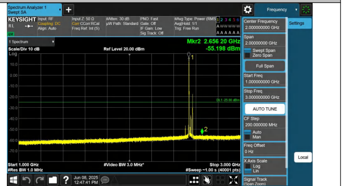
7-7-20MHz-15MHz-QPSK-QPSK-21201-21372-1RB#0-1RB#74-1 000~3000MHz-PASS
