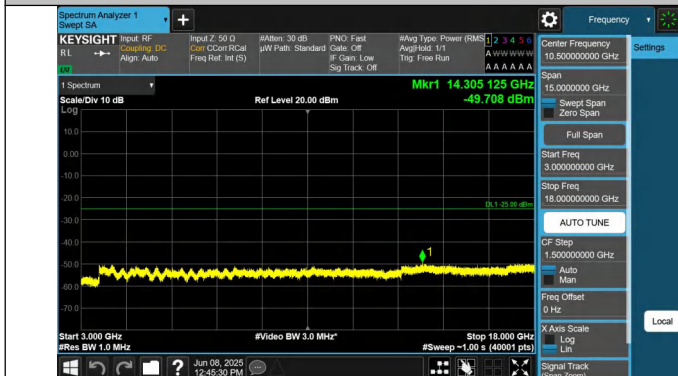
7-7-20MHz-15MHz-QPSK-QPSK-21026-21197-1RB#0-1RB#74-3 000~18000MHz-PASS
