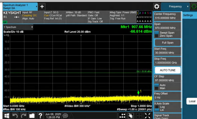
7-7-20MHz-20MHz-QPSK-QPSK-21001-21199-1RB#99-0RB#0-3 0~1000MHz-PASS
