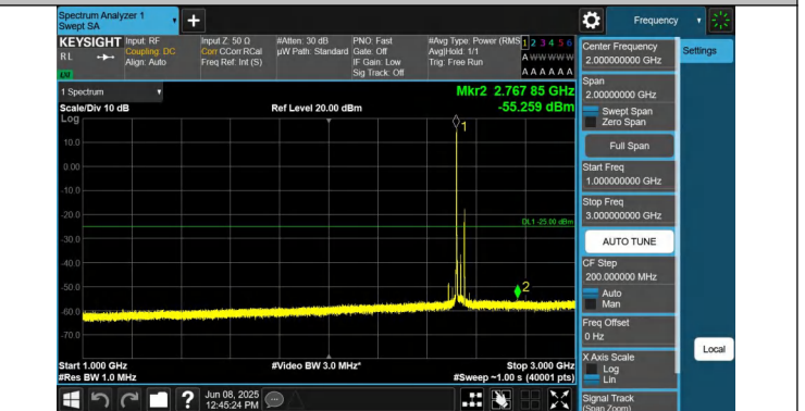
7-7-20MHz-15MHz-QPSK-QPSK-21026-21197-1RB#0-1RB#74-1 000~3000MHz-PASS
