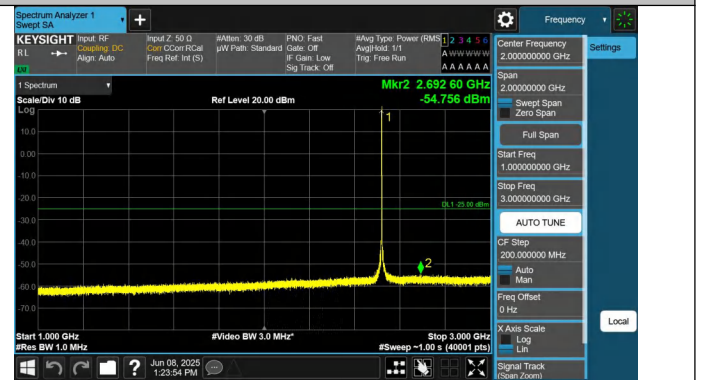
7-7-20MHz-20MHz-QPSK-QPSK-20850-21048-1RB#99-0RB#0-1000~3000MHz-PASS
