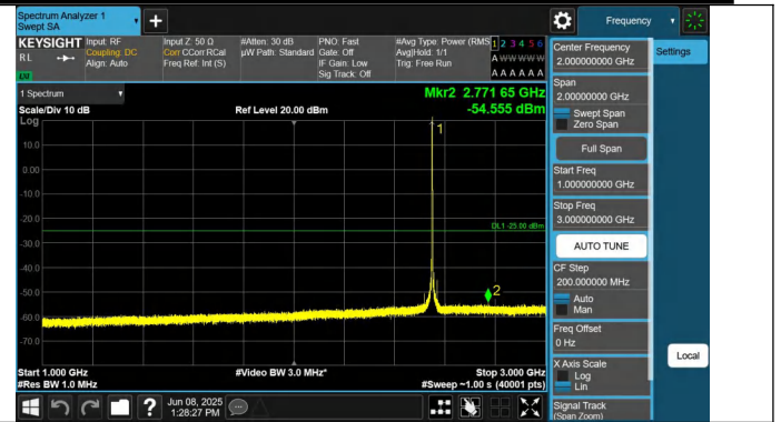
7-7-20MHz-20MHz-QPSK-QPSK-21152-21350-1RB#99-0RB#0-1 000~3000MHz-PASS
