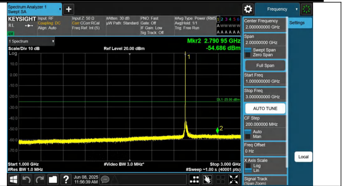
00~3000MHz-PASS
