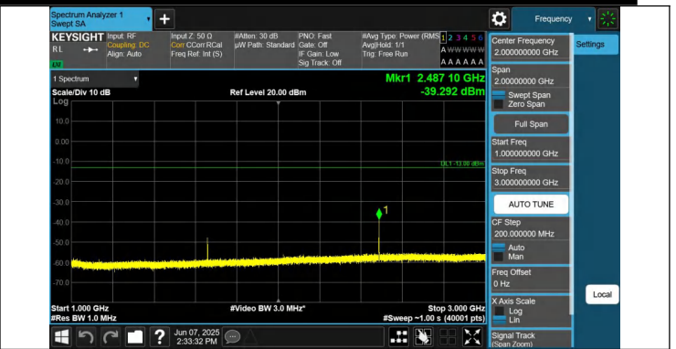
5-5-5MHz-10MHz-QPSK-QPSK-20428-20500-1RB#24-0RB#0-10 00~3000MHz-PASS
