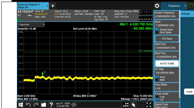
5-5-5MHz-10MHz-QPSK-QPSK-20428-20500-1RB#0-0RB#0-300 0~10000MHz-PASS
