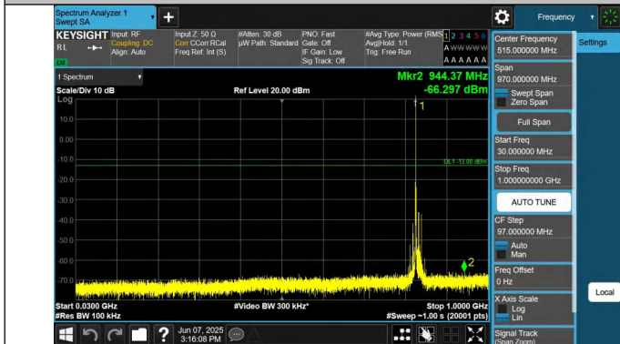
5-5-10MHz-5MHz-QPSK-QPSK-20500-20572-1RB#0-0RB#0-30~ 1000MHz-PASS
