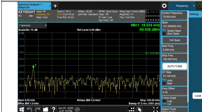
5-5-5MHz-10MHz-QPSK-QPSK-20528-20600-1RB#24-0RB#0-0. 009~0.15MHz-PASS
