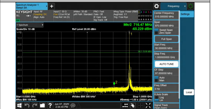
5-5-5MHz-10MHz-QPSK-QPSK-20478-20550-1RB#0-0RB#0-30~ 1000MHz-PASS
