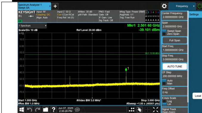
5-5-5MHz-10MHz-QPSK-QPSK-20478-20550-1RB#24-0RB#0-10 00~3000MHz-PASS
