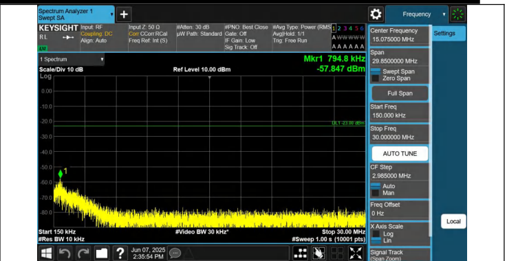
5-5-5MHz-10MHz-QPSK-QPSK-20478-20550-1RB#0-1RB#49-0. 15~30MHz-PASS
