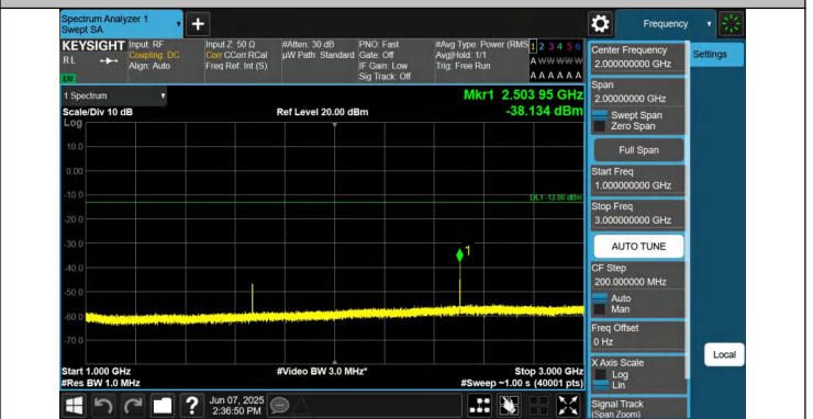
5-5-5MHz-10MHz-QPSK-QPSK-20528-20600-1RB#0-0RB#0-100 0~3000MHz-PASS
