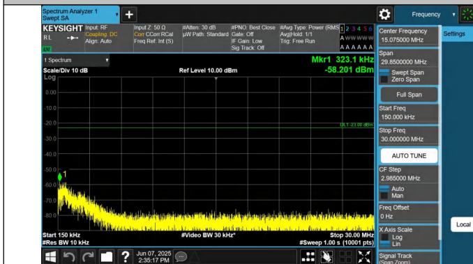
5-5-5MHz-10MHz-10MHz-QPSK-QPSK-20478-20550-1RB#24-0RB#0-0. 15~30MHz-PASS
