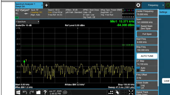
5-5-5MHz-10MHz-QPSK-QPSK-20528-20600-1RB#0-0RB#0-0.0 09~0.15MHz-PASS
