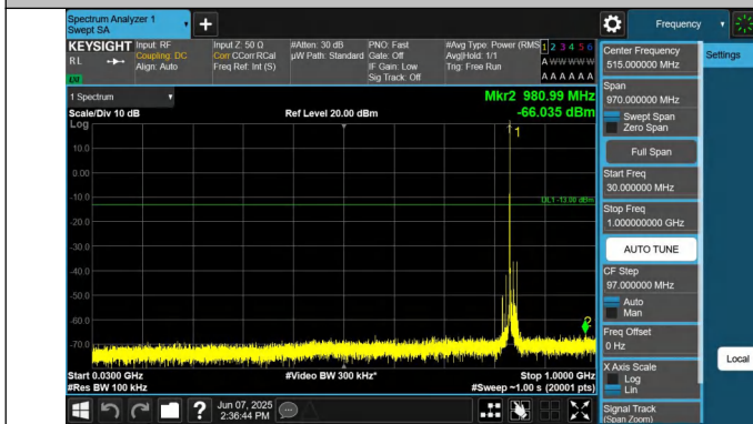
5-5-5MHz-10MHz-QPSK-QPSK-20528-20600-1RB#0-0RB#0-30~ 1000MHz-PASS
