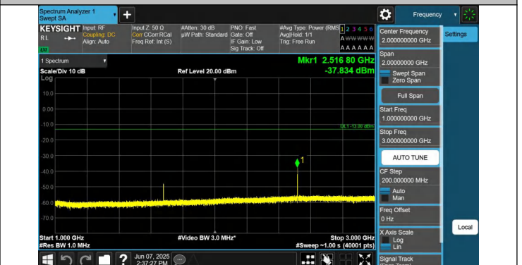
5-5-5MHz-10MHz-QPSK-QPSK-20528-20600-1RB#24-0RB#0-10 00~3000MHz-PASS
