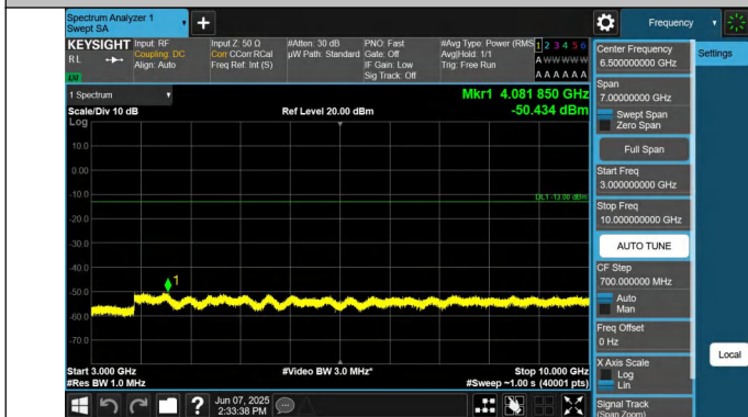
5-5-5MHz-10MHz-QPSK-QPSK-20428-20500-1RB#24-0RB#0-30 00~10000MHz-PASS
