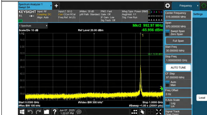
5-5-3MHz-5MHz-QPSK-QPSK-20586-20625-1RB#0-0RB#0-30~1 000MHz-PASS
