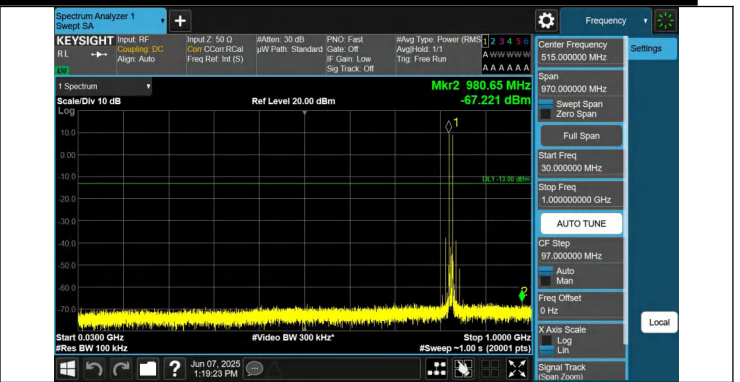
5-5-3MHz-5MHz-QPSK-QPSK-20416-20455-1RB#0-1RB#24-30~ 1000MHz-PASS
