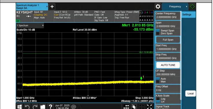
5-5-5MHz-3MHz-QPSK-QPSK-20425-20464-1RB#0-1RB#15-100 0~3000MHz-PASS
