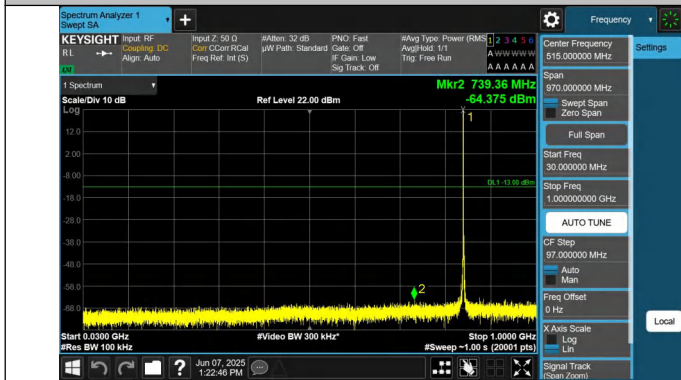
5-5-3MHz-5MHz-QPSK-QPSK-20586-20625-1RB#14-ORB#0-30~ 1000MHz-PASS
