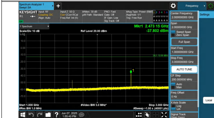
5-5-5MHz-3MHz-QPSK-QPSK-20425-20464-1RB#0-0RB#0-1000 ~3000MHz-PASS
