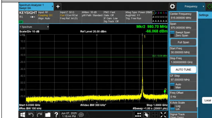
5-5-3MHz-5MHz-QPSK-QPSK-20416-20455-1RB#14-0RB#0-30~ 1000MHz-PASS
