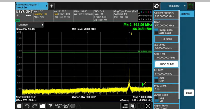
5-5-5MHz-3MHz-QPSK-QPSK-20425-20464-1RB#24-0RB#0-30~ 1000MHz-PASS
