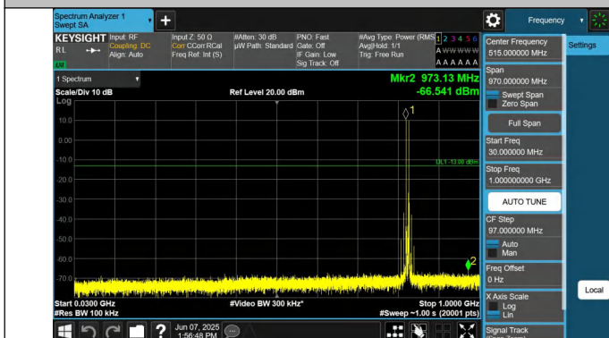
5-5-5MHz-3MHz-QPSK-QPSK-20425-20464-1RB#0-1RB#15-30~ 1000MHz-PASS
