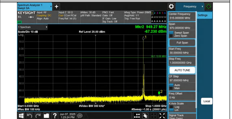
5-5-3MHz-5MHz-QPSK-QPSK-20586-20625-1RB#0-1RB#24-30~ 1000MHz-PASS
