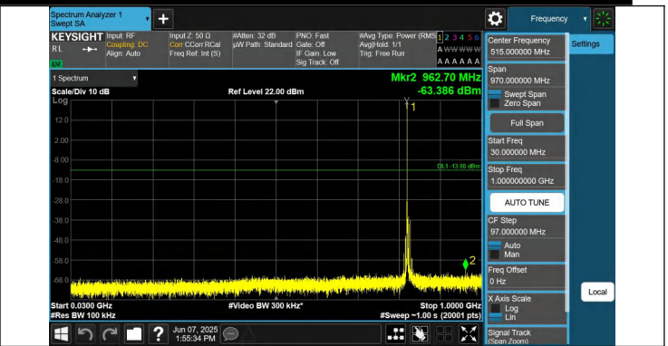
5-5-5MHz-3MHz-QPSK-QPSK-20425-20464-1RB#0-0RB#0-30~1 000MHz-PASS
