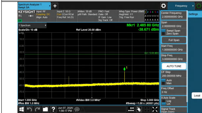
5-5-5MHz-3MHz-QPSK-QPSK-20425-20464-1RB#24-0RB#0-100 0~3000MHz-PASS
