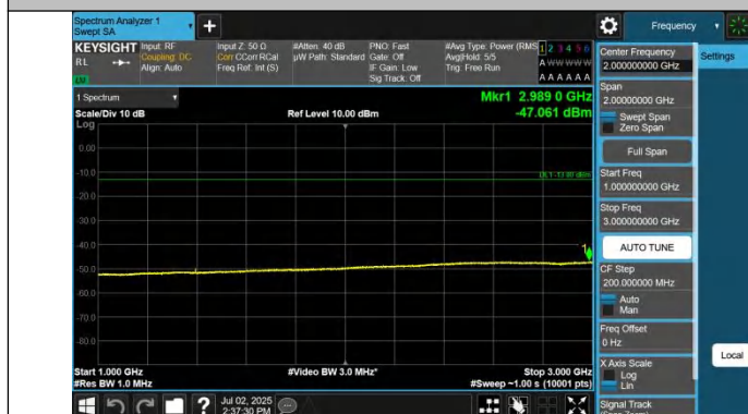
Band71-20MHz-QPSK-133372-1RB#99-1000~3000-PASS
