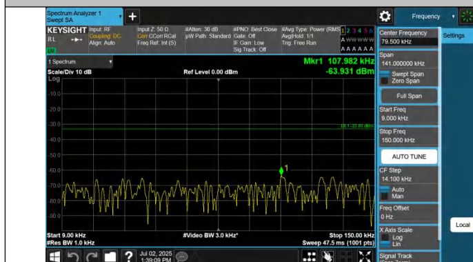
Band71-20MHz-QPSK-133372-1RB#0-0.009~0.15-PASS
