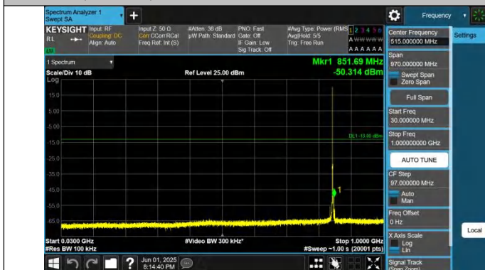
Band26(824-849)-3MHz-QPSK-27025-1RB#0-30~1000-PASS
