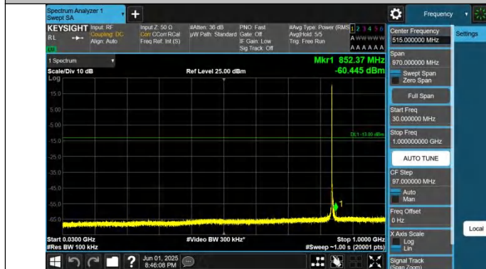
Band26(824-849)-10MHz-QPSK-26990-1RB#0-30~1000-PASS
