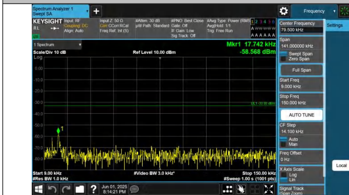
Band26(824-849)-3MHz-QPSK-27025-1RB#0-0.009~0.15-PASS
