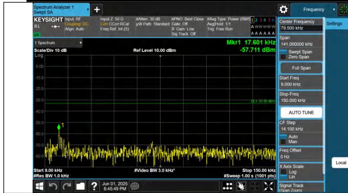
Band26(824-849)-10MHz-QPSK-26990-1RB#0-0.009~0.15-PASS
