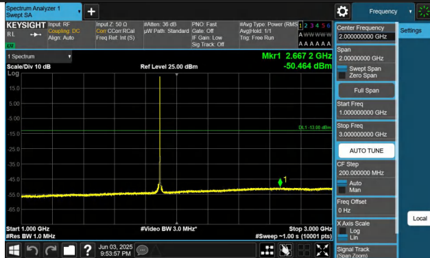
Band25-20MHz-QPSK-26365-1RB#99-1000~3000-PASS
