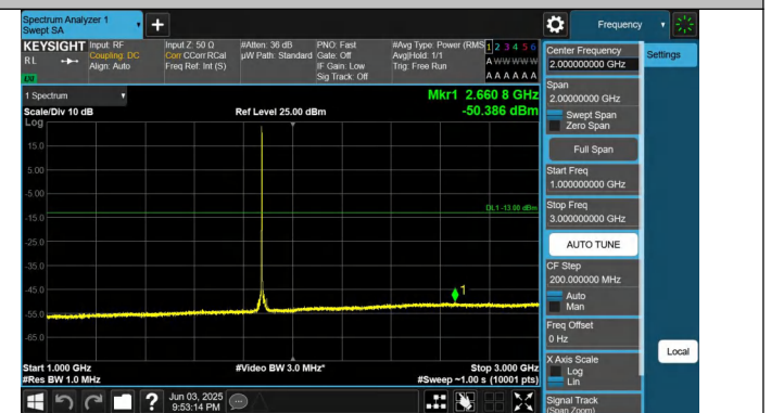
Band25-20MHz-QPSK-26365-1RB#0-1000~3000-PASS
