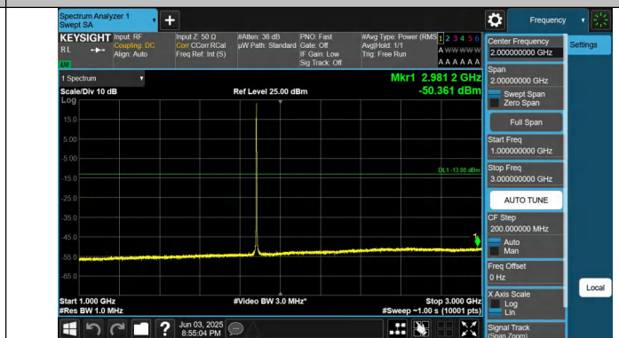
Band25-3MHz-QPSK-26365-1RB#0-1000~3000-PASS
