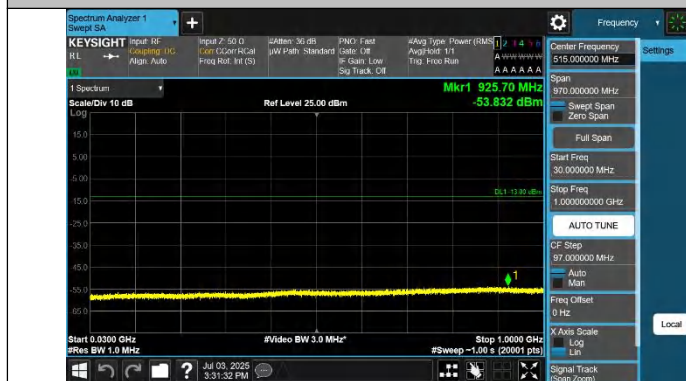
Band2-9400-3-30~1000MHz-PASS
