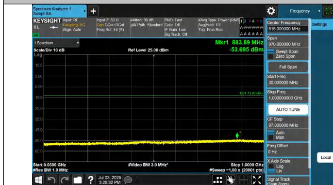
Band2-9400-1-30~1000MHz-PASS
