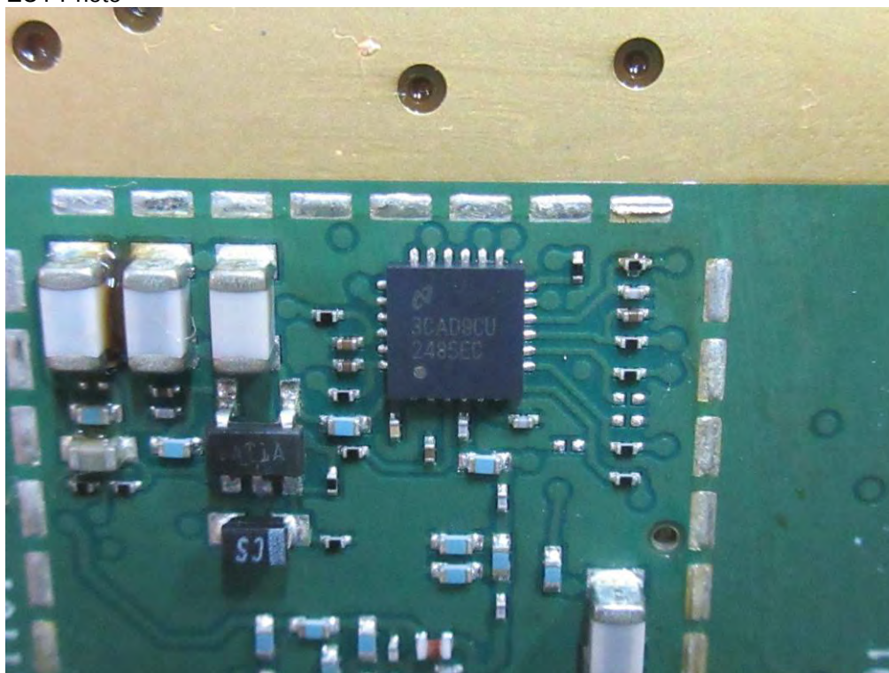
(94) EUT Photo
