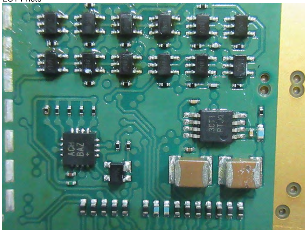
(96) EUT Photo
