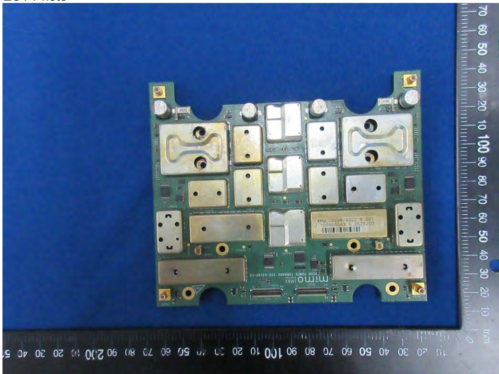
(54) EUT Photo
