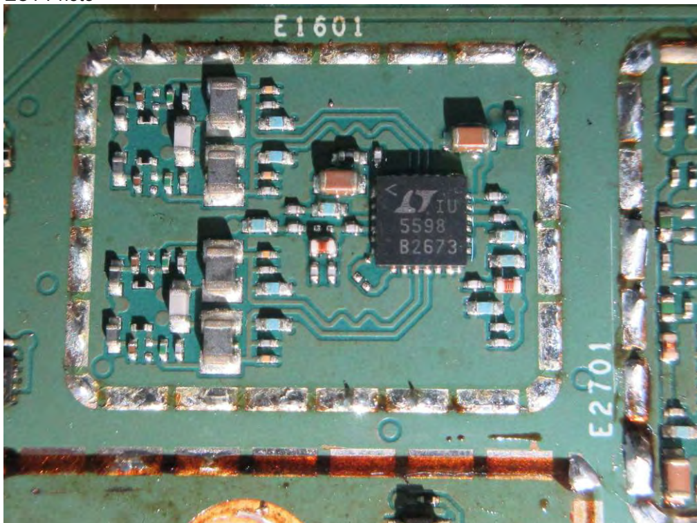
(62) EUT Photo
