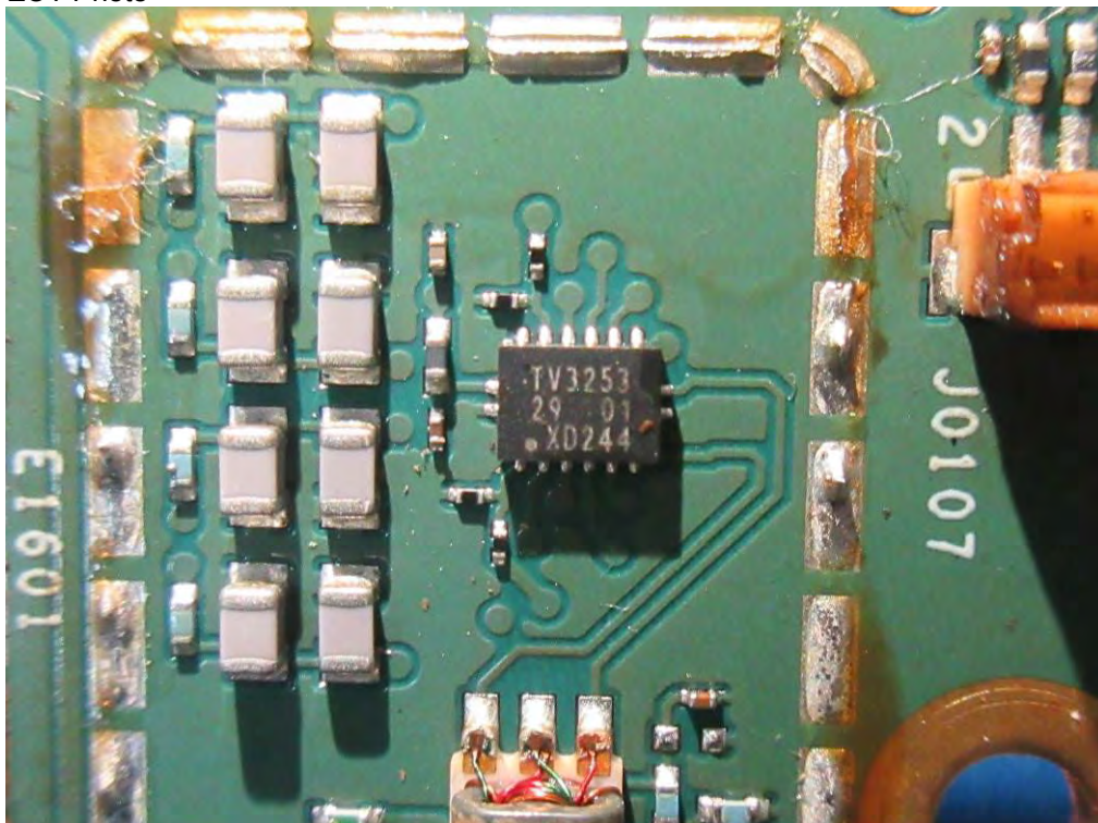
(66) EUT Photo
