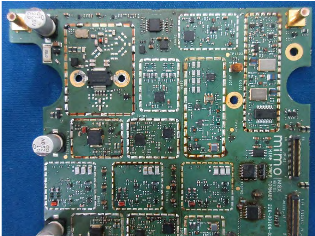
(56) EUT Photo
