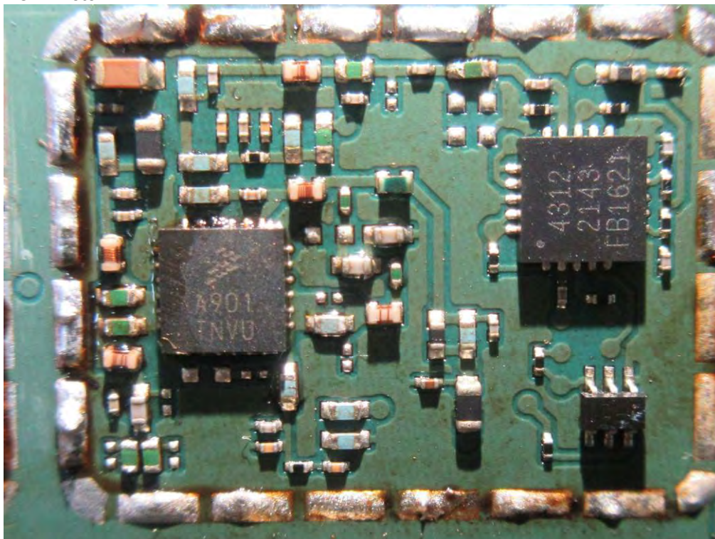
(64) EUT Photo
