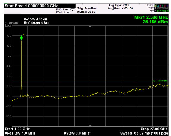
AWGN SIGNAL, 1GHz-27GHz
