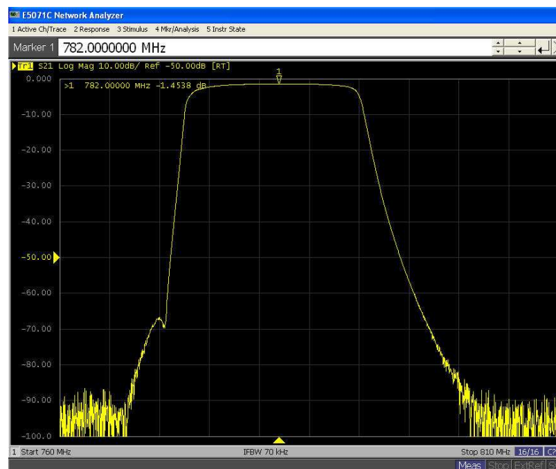
Up-link
