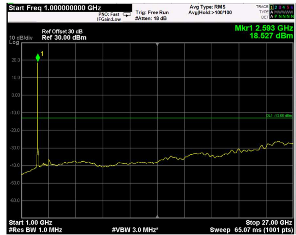
AWGN SIGNAL, 1GHz-27GHz
