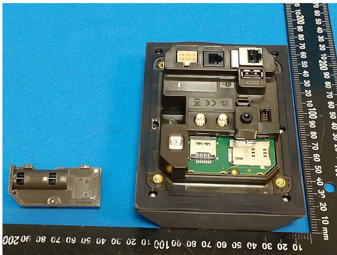
Configuration 2#(HVIN:AXIUM SX5000 CL/Eth/4G/WiFi/BT)
