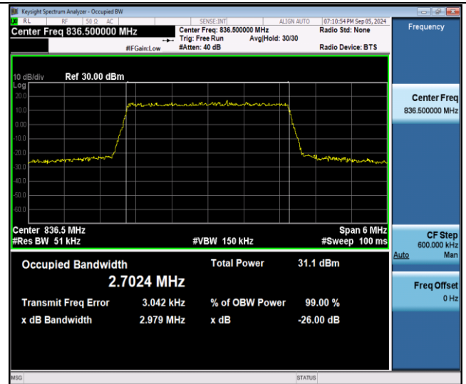
Band26(824-849)-3MHz-QPSK-26915-15RB#0-PASS
