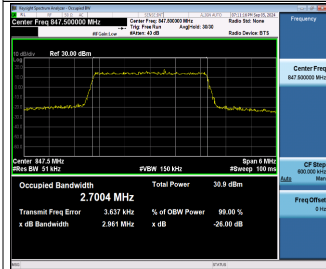
Band26(824-849)-3MHz-QPSK-27025-15RB#0-PASS
