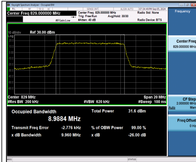
Band26(824-849)-10MHz-QPSK-26840-50RB#0-PASS
