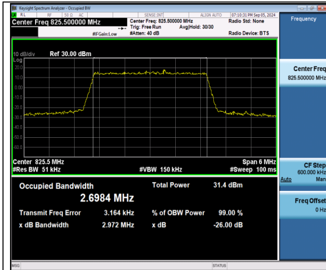
Band26(824-849)-3MHz-QPSK-26805-15RB#0-PASS
