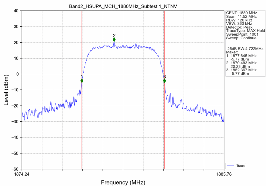
Band2_HSUPA_MCH_1880MHz_Subtest 1_NTNV
