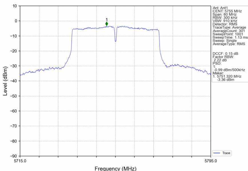
802.11ac(VHT40)_LCH_5755MHz_Ant1_NTNV
