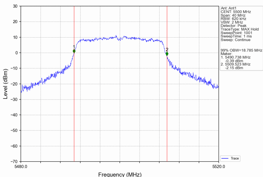
802.11ac(VHT20)_LCH_5500MHz_Ant1_NTNV
