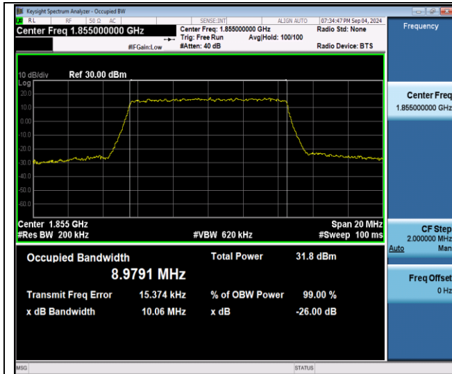
Band2-10MHz-QPSK-18650-50RB#0-PASS
