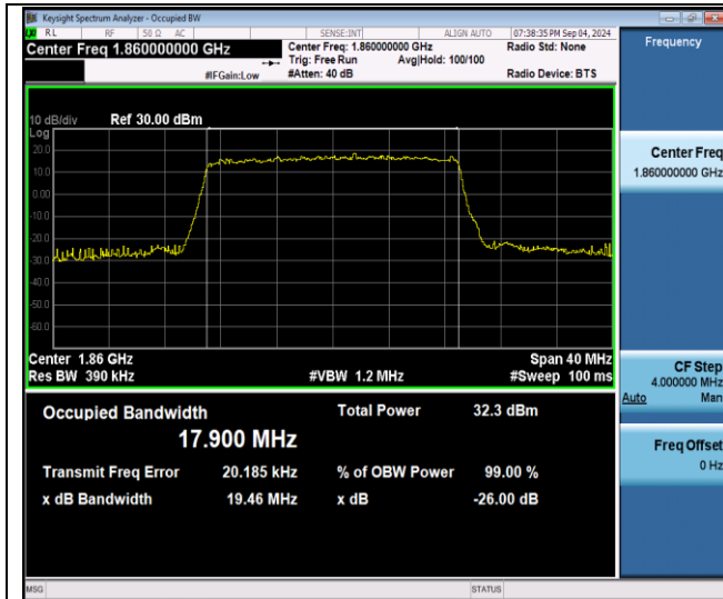
Band2-20MHz-QPSK-18700-100RB#0-PASS
