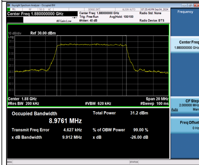
Band2-10MHz-16QAM-18900-50RB#0-PASS
