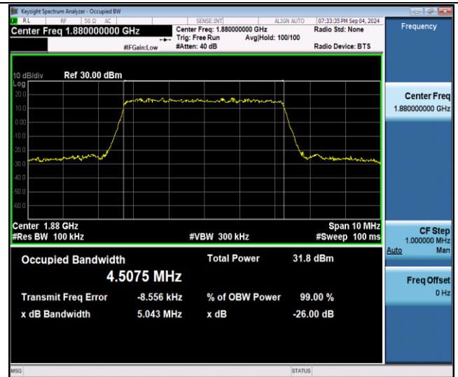
Band2-5MHz-QPSK-18900-25RB#0-PASS
