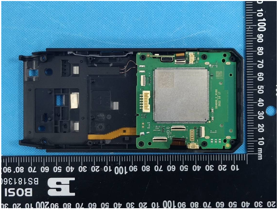
NFC Antenna
