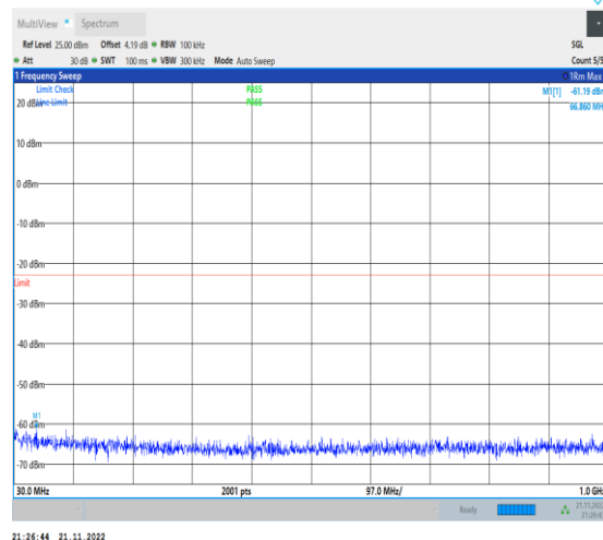
1-N70-PC3-15-15-M-1-DFT-PI2BPSK-Inner_1RB_Le ft-1@1-30-1000-Ant1-66.86--61.19--23-PASS
