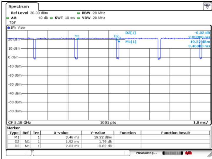
802.11n_HT20
