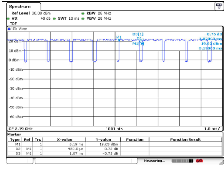
802.11n_HT40
