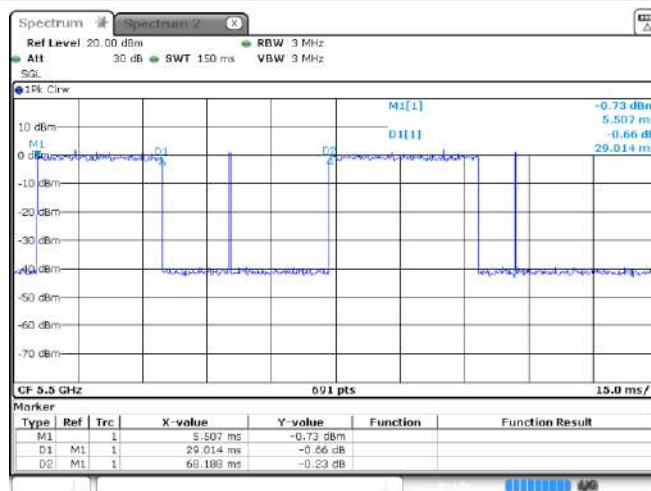
11a 5500 MHz
