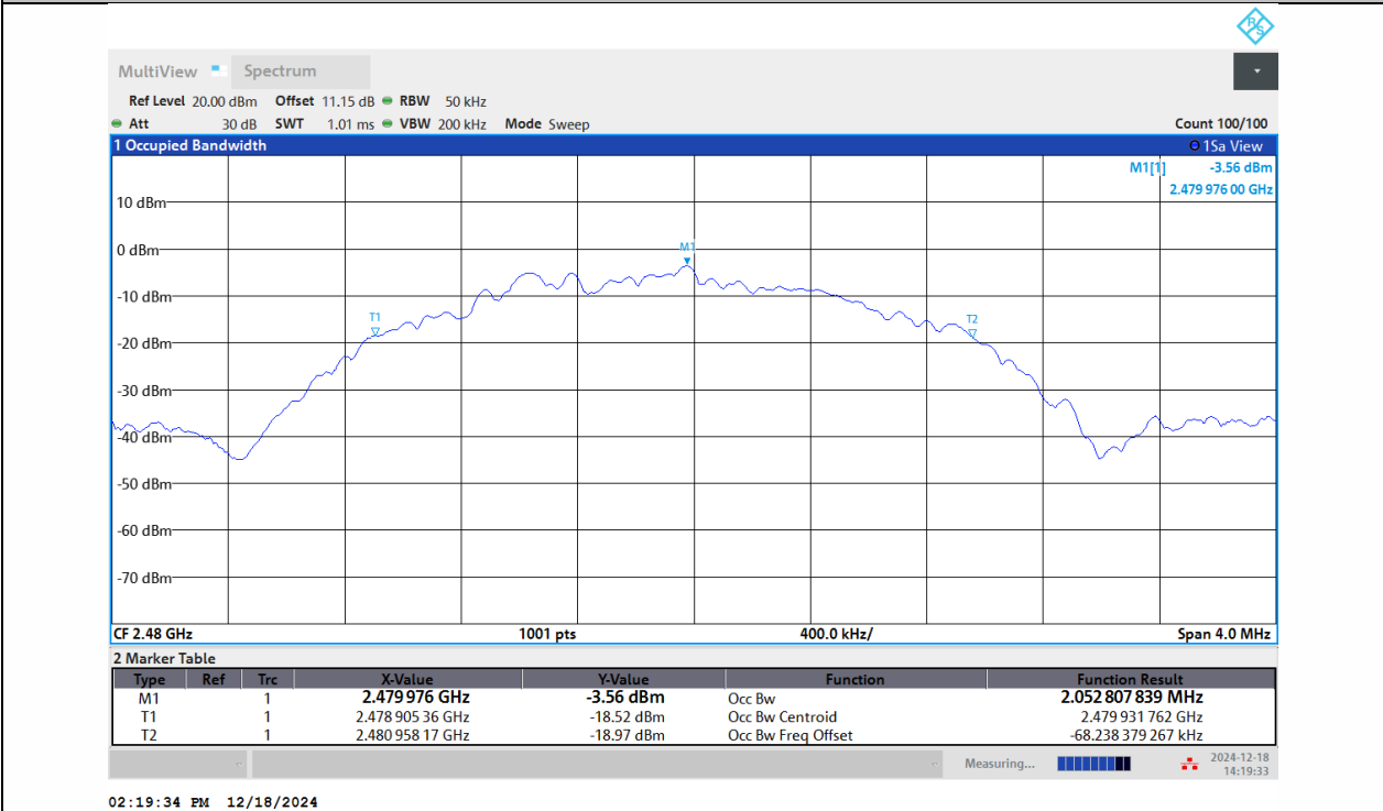
BLE_2M-Ant1-2480
