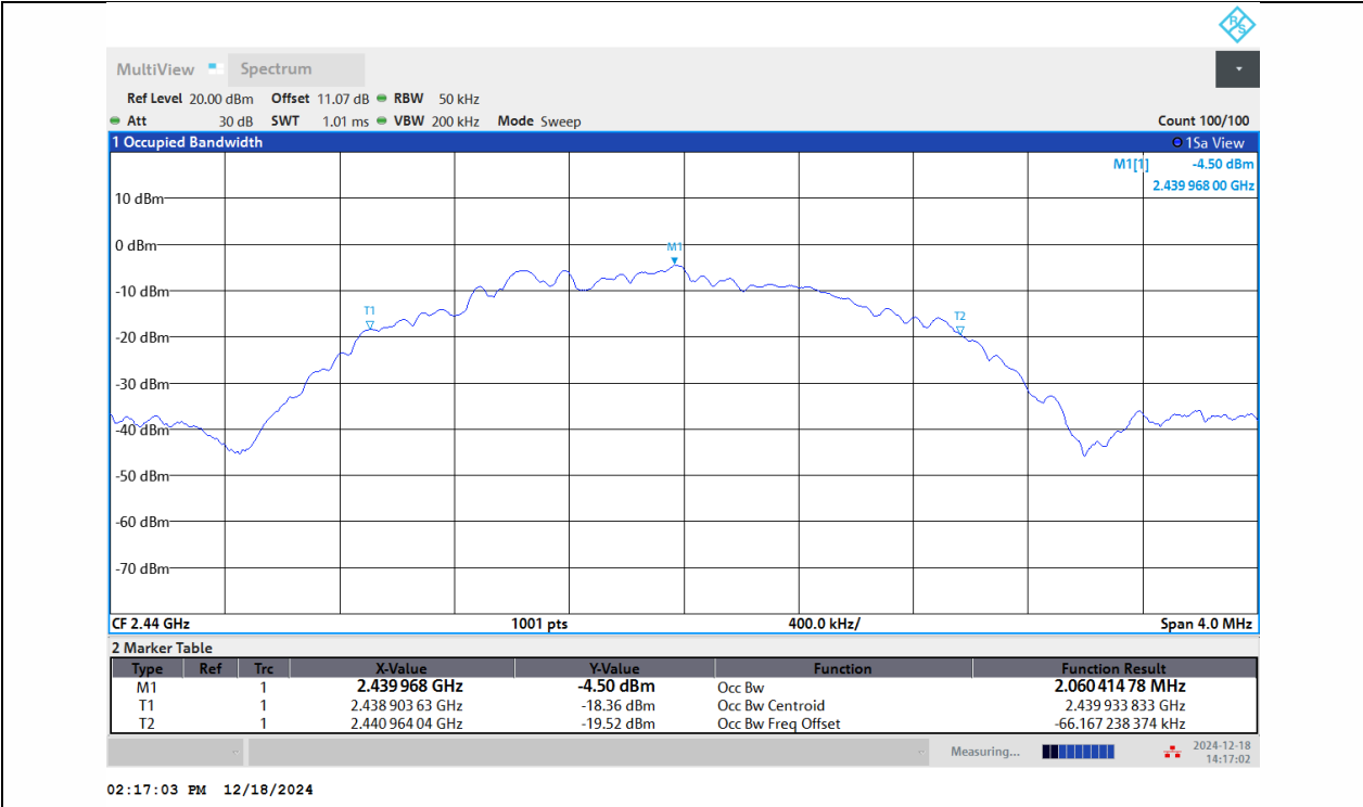
BLE_2M-Ant1-2440
