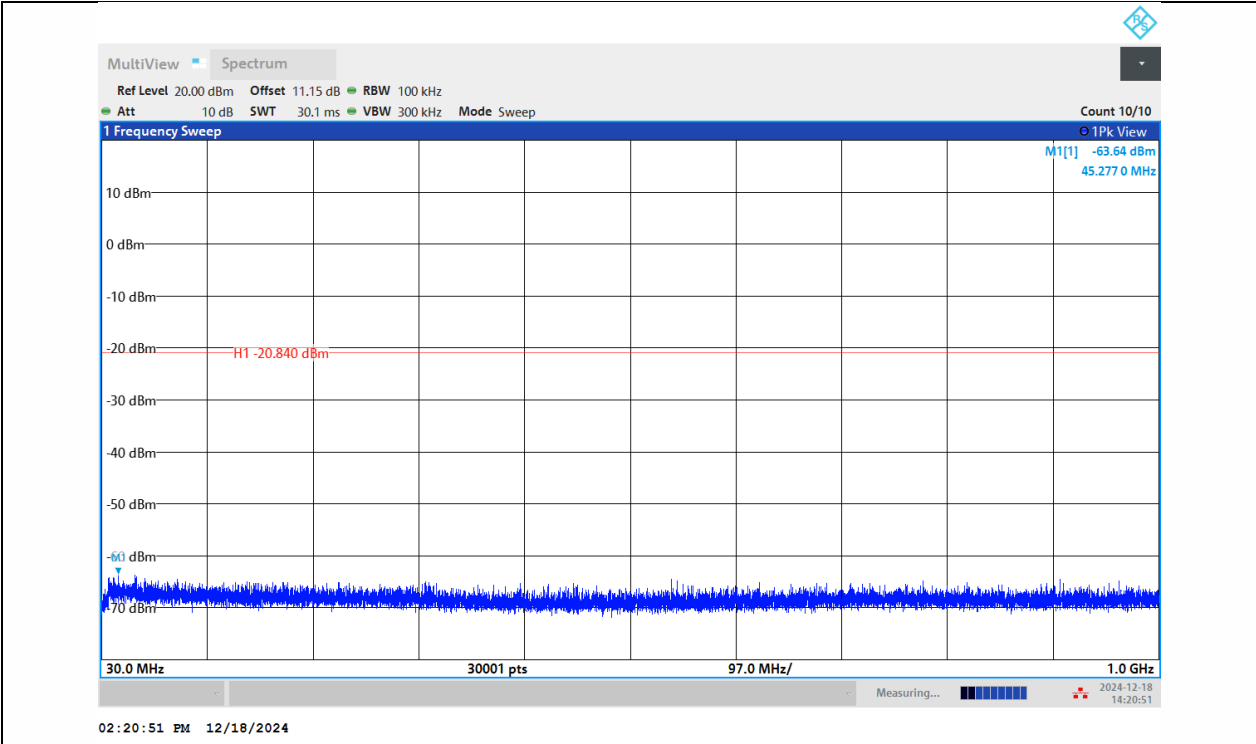
BLE_2M-Ant1-2480-30~1000-PASS
