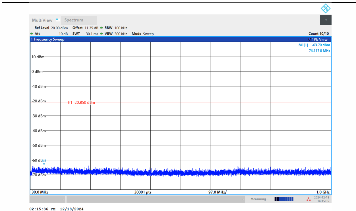
BLE_2M-Ant1-2402-30~1000-PASS
