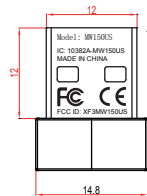
正面
