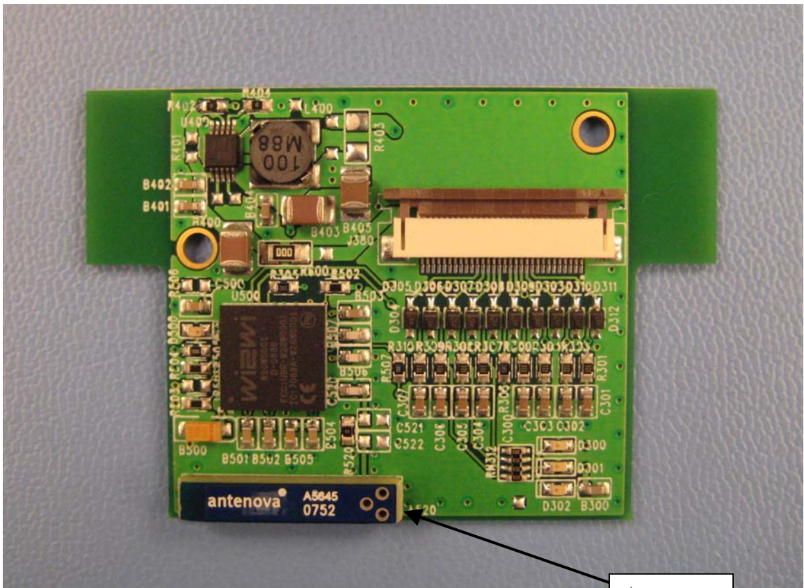
Antenna
