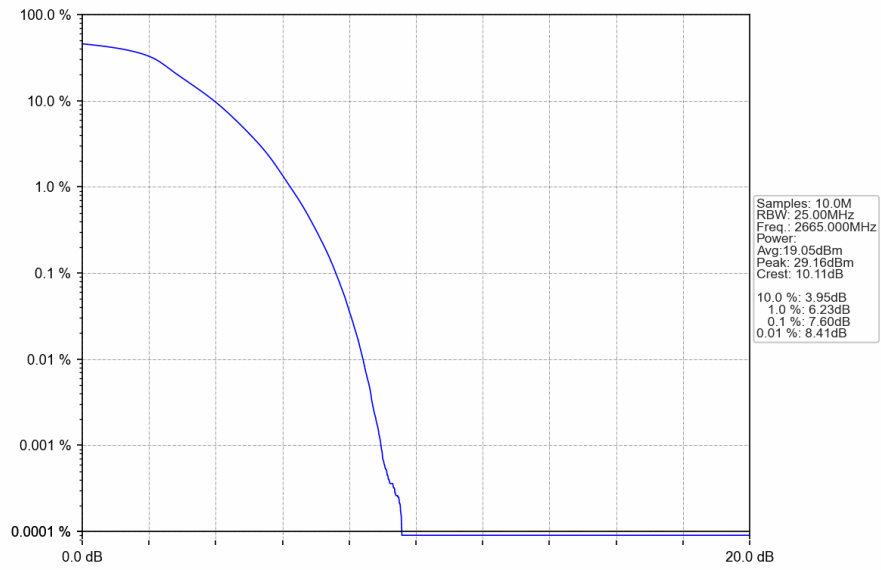
Band41_20MHz_QPSK_HCH_2665MHz_RB_100_0_NTNV
