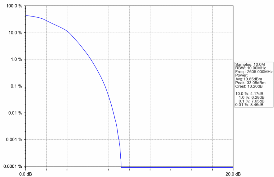
Band41_10MHz_16QAM_MCH_2605MHz_RB_50_0_NTNV
