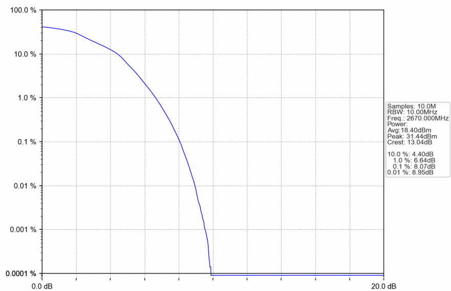
Band41_10MHz_16QAM_HCH_2670MHz_RB_50_0_NTNV
