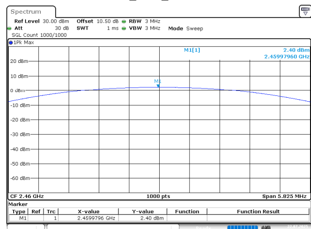
3EDR_DH1_2460MHz
