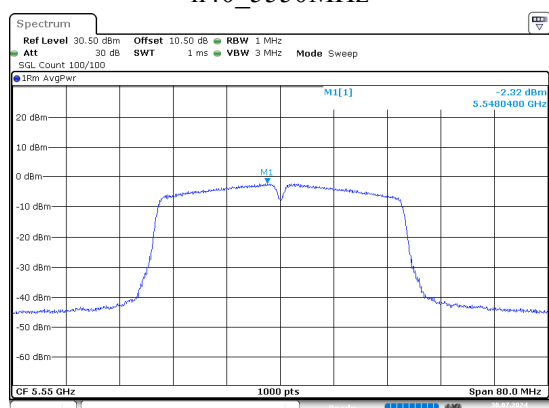
n40_5550MHz
