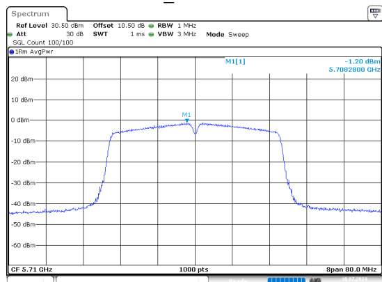
n40_5710MHz
