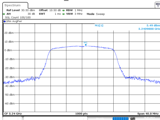
a_5240MHz
