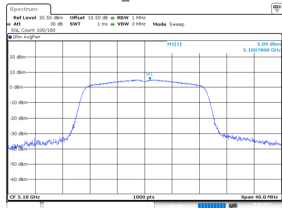
n20_5180MHz
