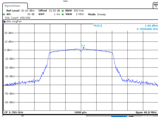
a_5785MHz
