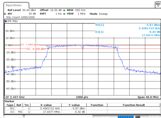
802.11n20_2437MHz
