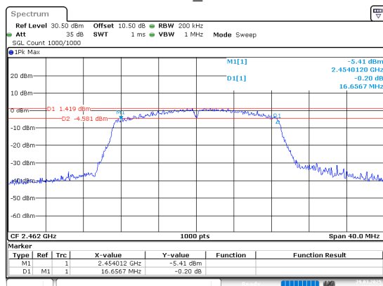
802.11n20_2462MHz
