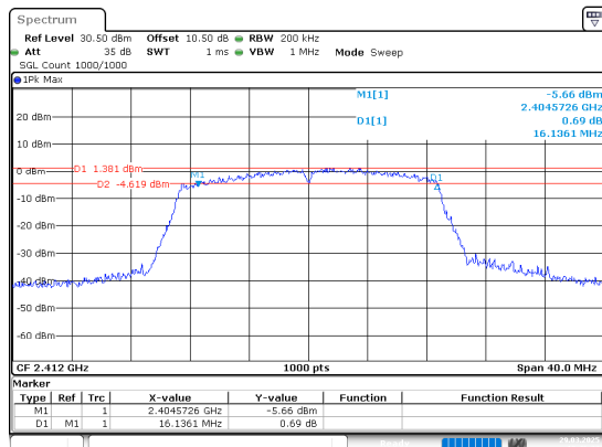
802.11n20_2412MHz
