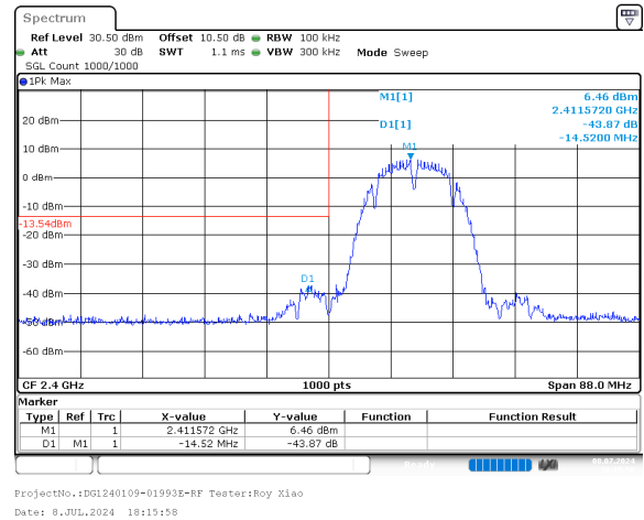
b_2412MHz_Chain 0
