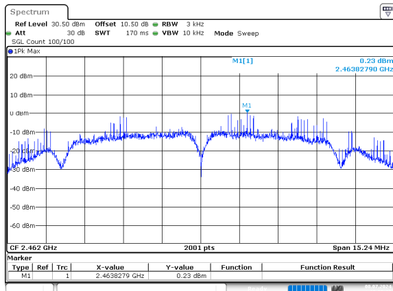
b_2462MHz_Chain 0
