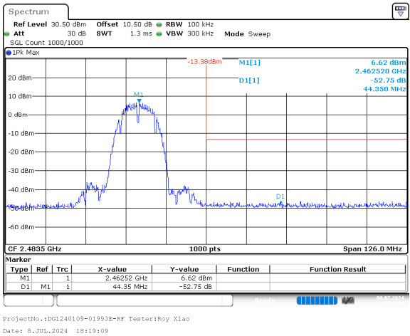
b_2462MHz_Chain 0
