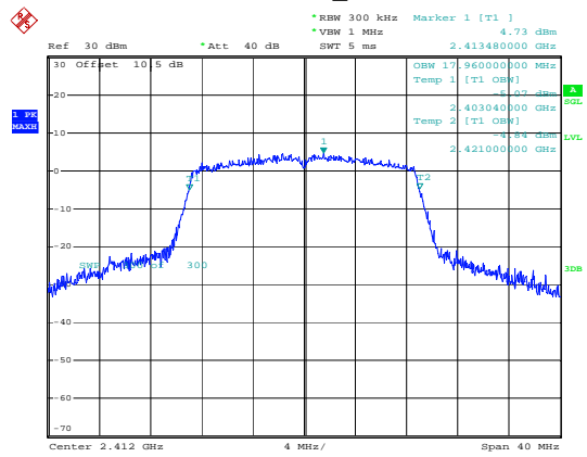
802.11n20_2412MHz
