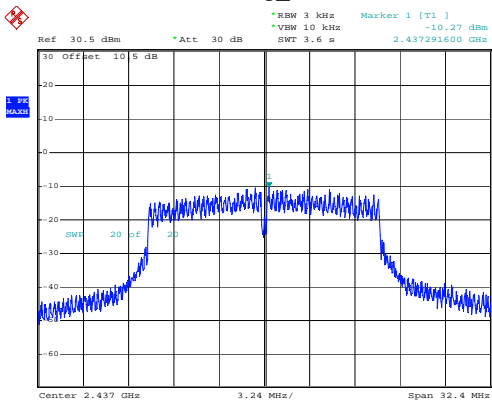
802.11g_2437MHz
