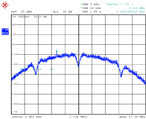
802.11b_2462MHz
