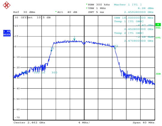
802.11n20_2462MHz
