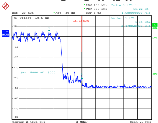
2EDR_2DH1_Hopping_Upper
