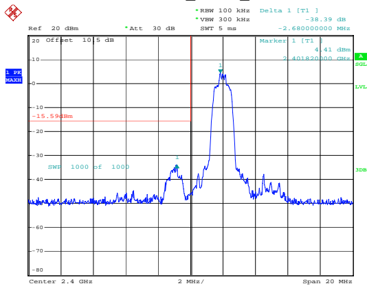
2EDR_2DH1_Low
