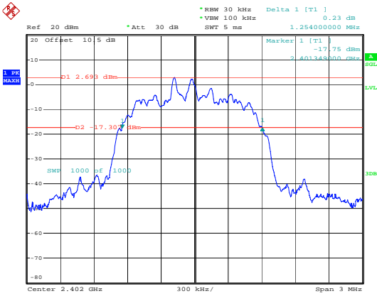
2EDR_2DH1_Low
