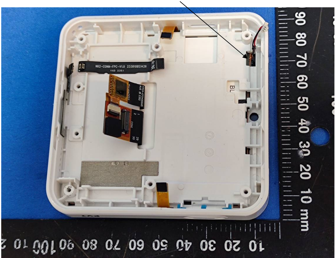
NFC Antenna
