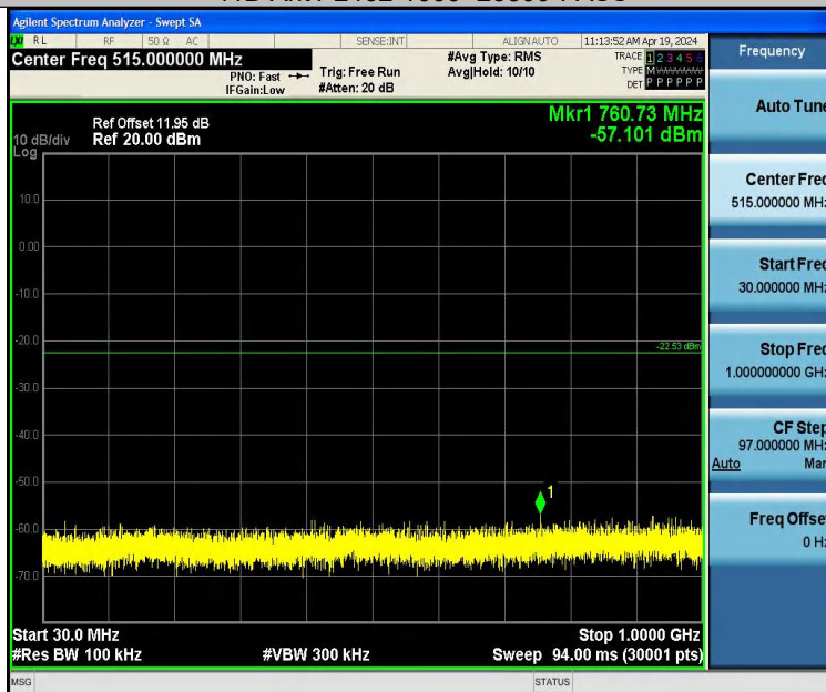
11G-Ant1-2412-30~1000-PASS
