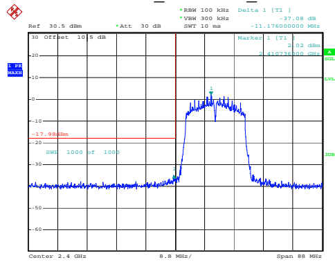
802.11n20_2412MHz_Chain 1
