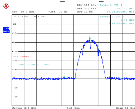
802.11b_2412MHz_Chain 1
