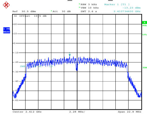
802.11n20_2412MHz_Chain 0
