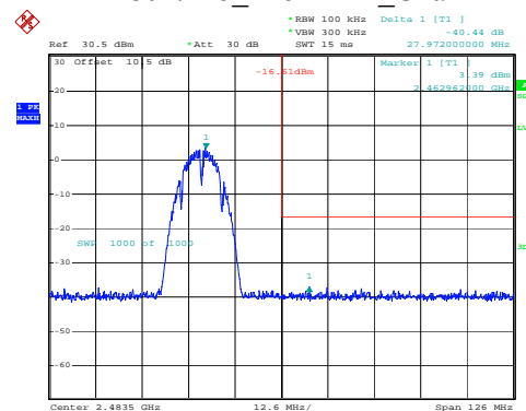
802.11b_2462MHz_Chain 1
