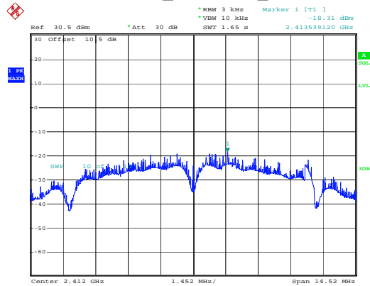
802.11b_2412MHz_Chain 0
