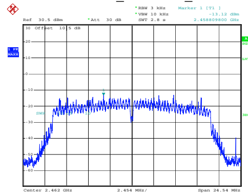
802.11n20_2462MHz_Chain 1
