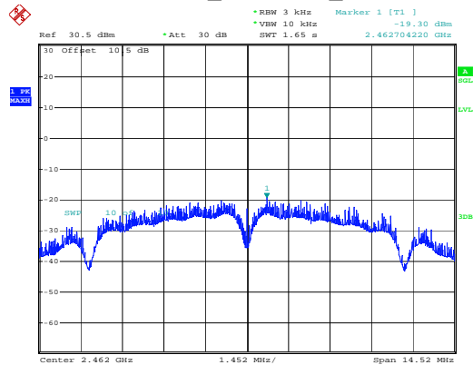
802.11b_2462MHz_Chain 0
