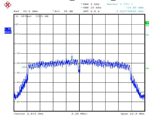
802.11n20_2412MHz_Chain 1
