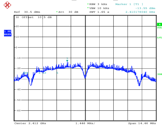
802.11b_2412MHz_Chain 1
