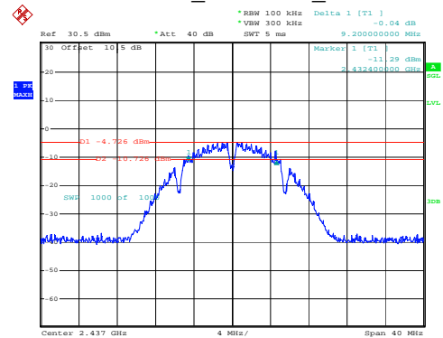
802.11b_2437MHz_Chain 0
