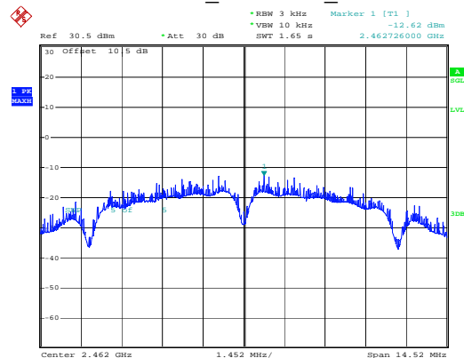
802.11b_2462MHz_Chain 1
