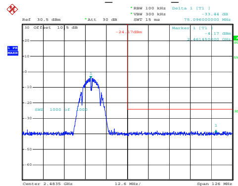
802.11b_2462MHz_Chain 0
