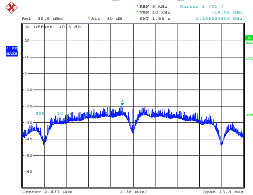
802.11b_2437MHz_Chain 0
