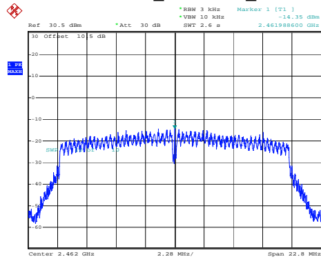
802.11n20_2462MHz_Chain 0
