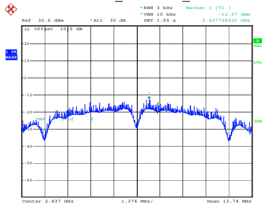
802.11b_2437MHz_Chain 1
