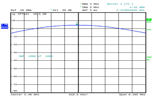
\pi/4 -DQPSK_High
