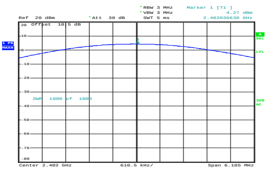
\pi/4 -DQPSK_Low
