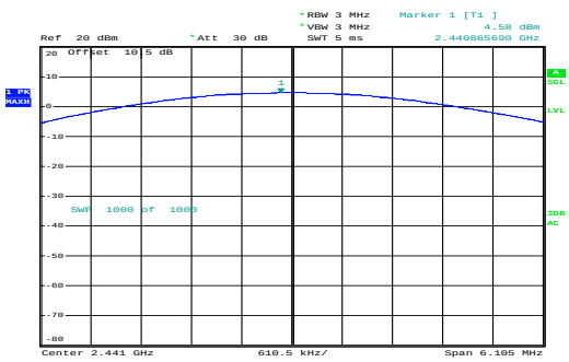
\pi/4 -DQPSK_Middle
