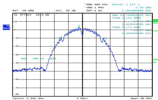
b_2462MHz_Chain 0
