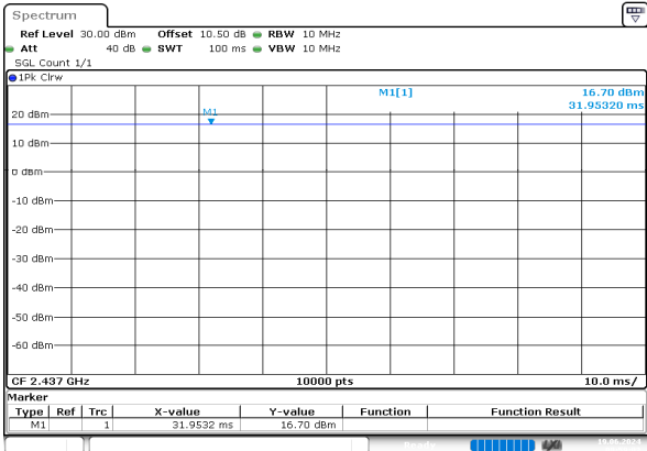
b_2437MHz_Chain 0
