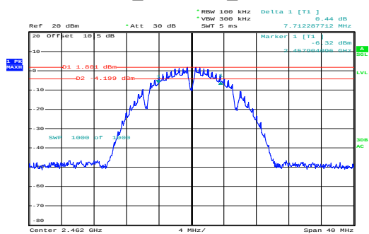
b_2462MHz_Chain 0
