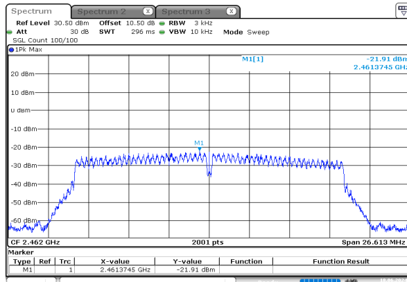
n20_2462MHz_Chain 0
