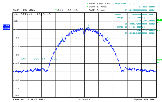
b_2412MHz_Chain 0
