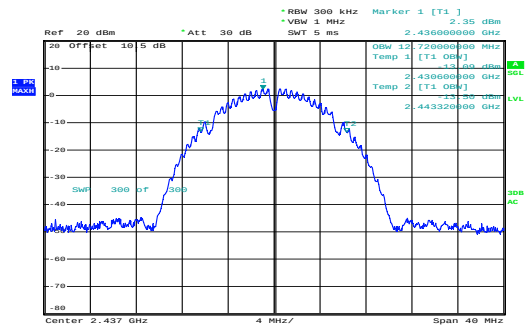
b_2437MHz_Chain 0
