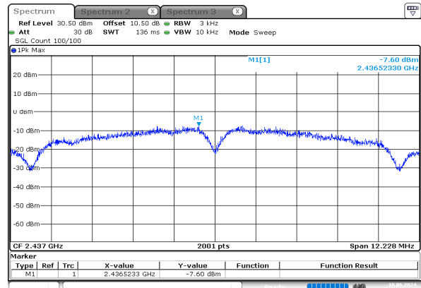
b_2437MHz_Chain 0
