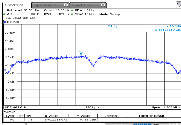
b_2462MHz_Chain 0
