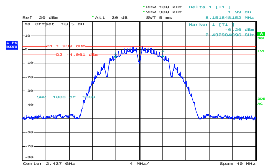
b_2437MHz_Chain 0
