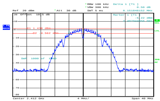
b_2412MHz_Chain 0
