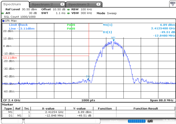
b_2412MHz_Chain 0
