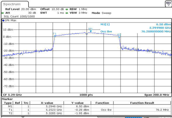
ac80_5290MHz_Chain 0
