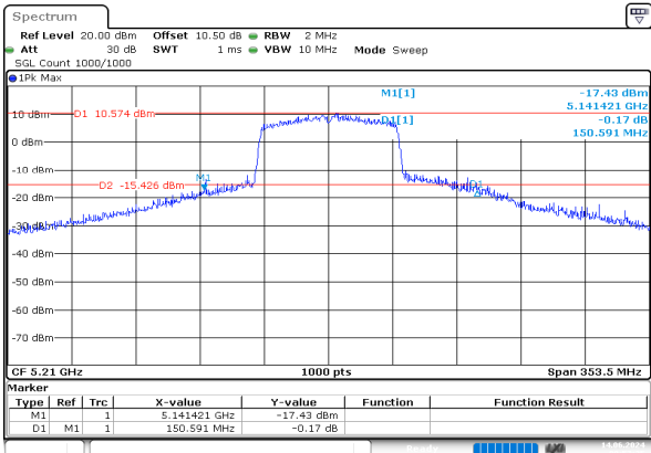
ac80_5210MHz_Chain 0
