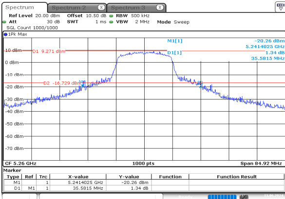
a_5260MHz_Chain 0
