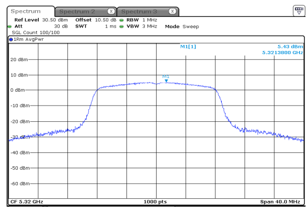
a_5320MHz_Chain 0
