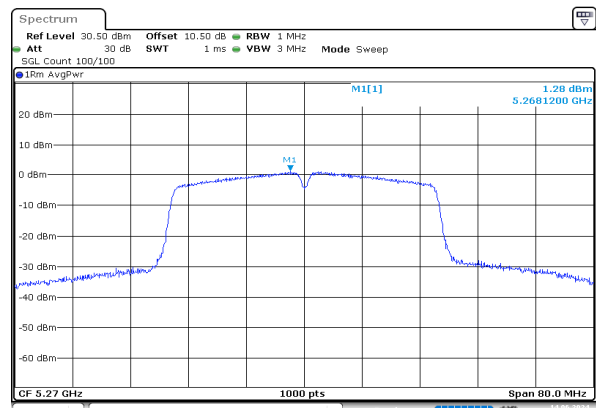
n40_5270MHz_Chain 0
