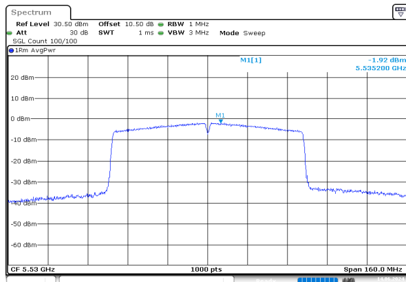
ac80_5530MHz_Chain 0
