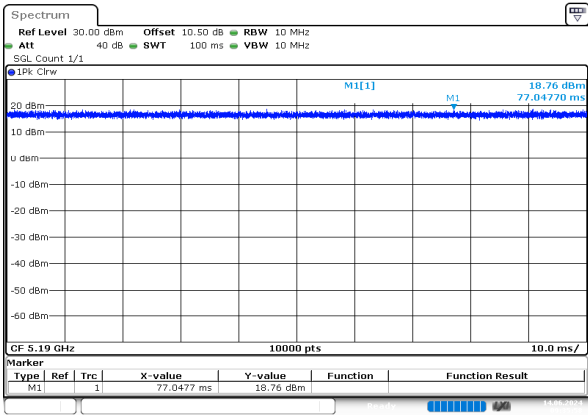
n40_5190MHz_Chain 0
