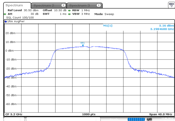
a_5200MHz_Chain 0
