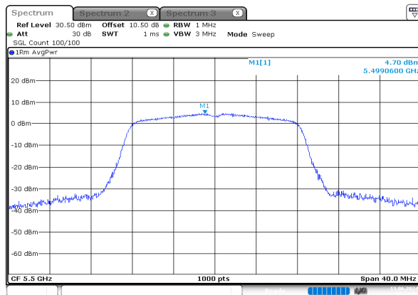
a_5500MHz_Chain 0
