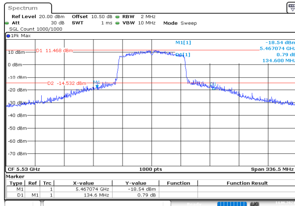
ac80_5530MHz_Chain 0
