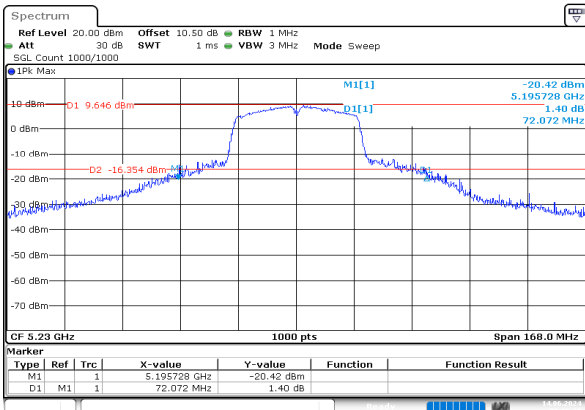
n40_5230MHz_Chain 0
