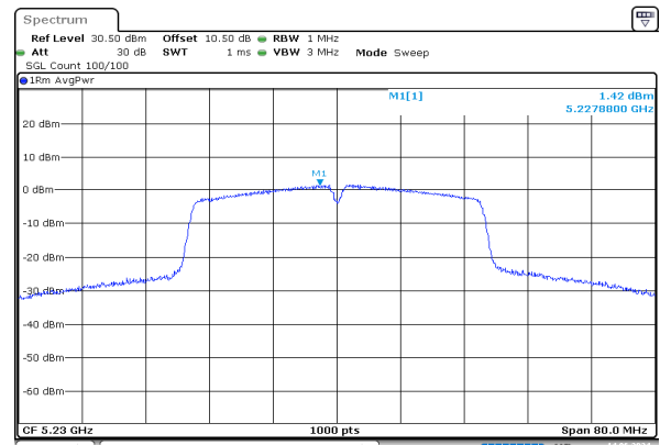
n40_5230MHz_Chain 0
