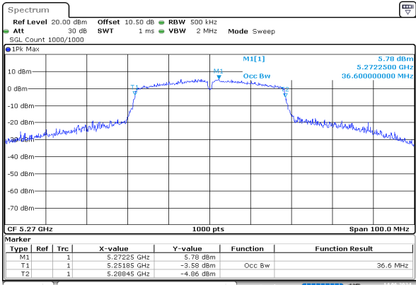
n40_5270MHz_Chain 0
