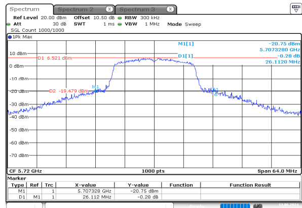
n20_5720MHz_Chain 0
