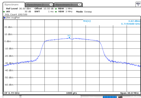
a_5720MHz_Chain 0
