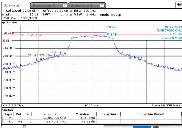
a_5320MHz_Chain 0
