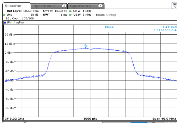
n20_5320MHz_Chain 0
