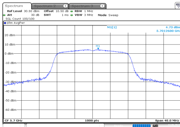
a_5700MHz_Chain 0
