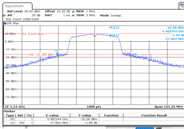
n40_5510MHz_Chain 0
