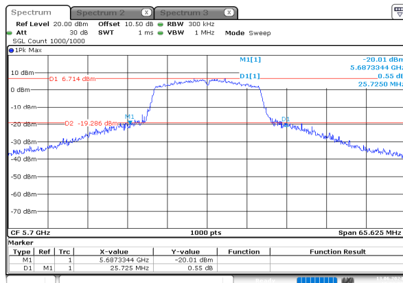
n20_5700MHz_Chain 0
