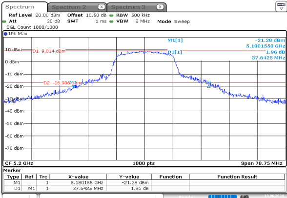
a_5200MHz_Chain 0
