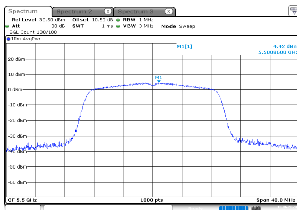
n20_5500MHz_Chain 0
