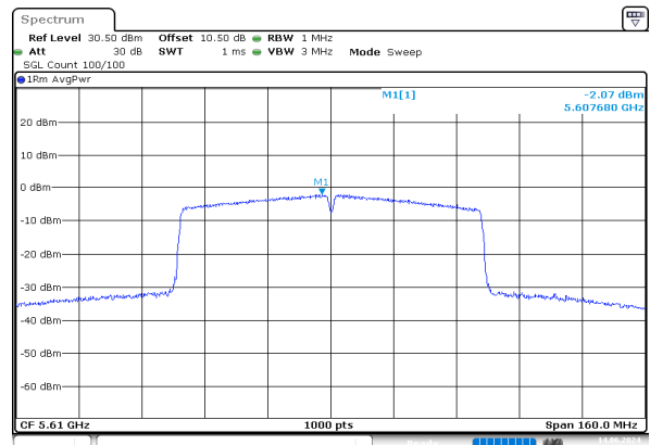
ac80_5610MHz_Chain 0
