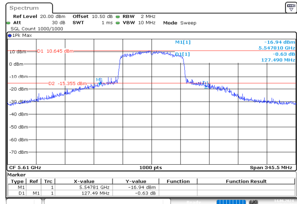
ac80_5610MHz_Chain 0
