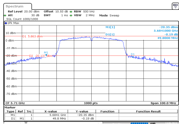
n40_5710MHz_Chain 0
