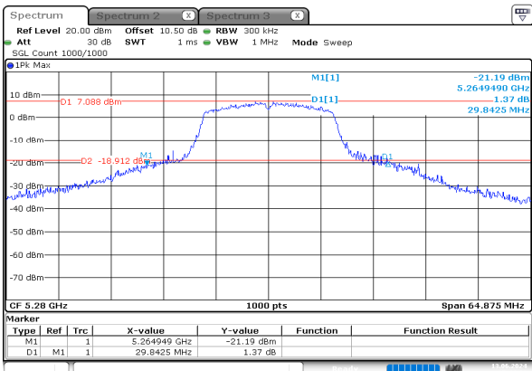
a_5280MHz_Chain 0
