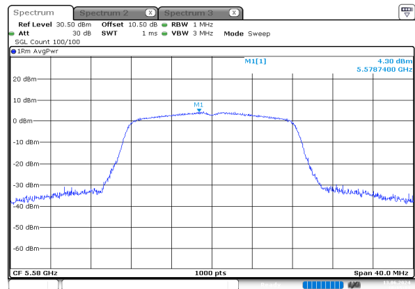
a_5580MHz_Chain 0
