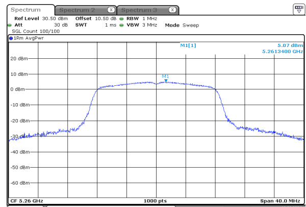
a_5260MHz_Chain 0
