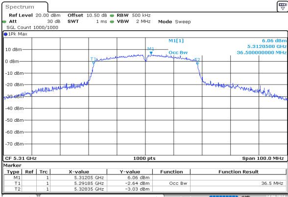
n40_5310MHz_Chain 0
