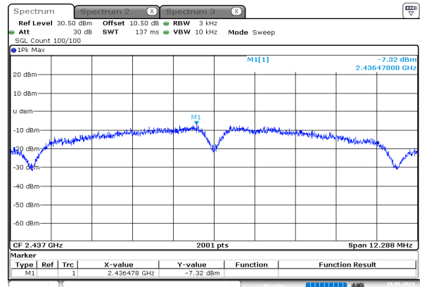
b_2437MHz_Chain 0
