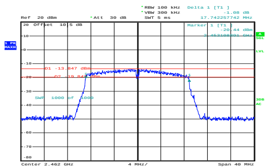
n20_2462MHz_Chain 0
