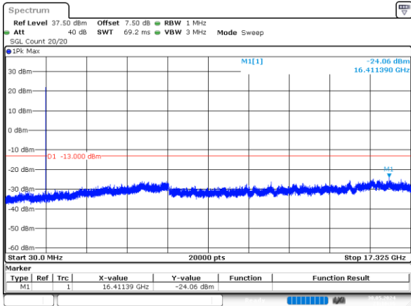
1.4MHz_Middle_QPSK_6@0 -24.06dBm
