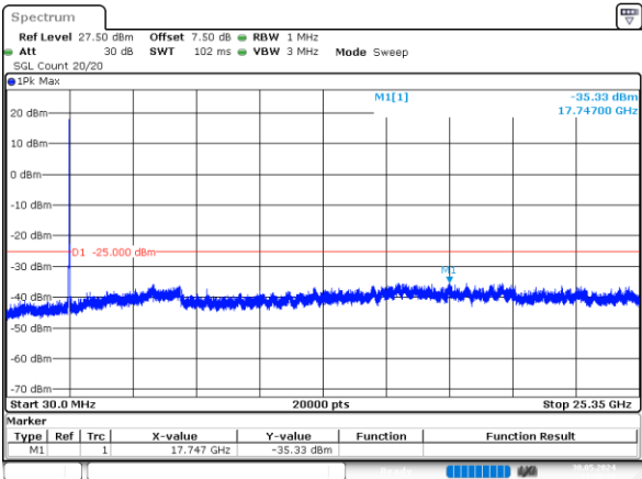
10MHz_Middle_QPSK_50@0 -35.33dBm
