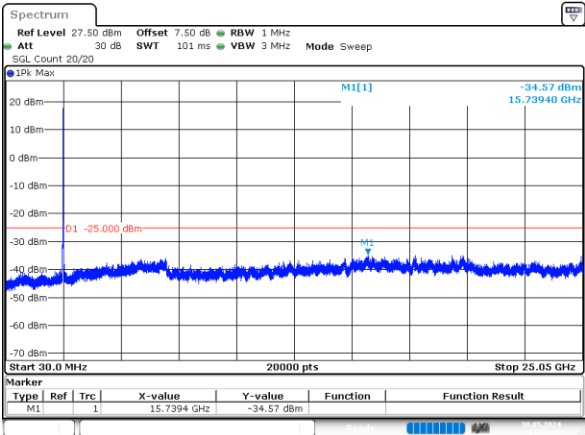
10MHz_Low_QPSK_50@0 -34.57dBm
