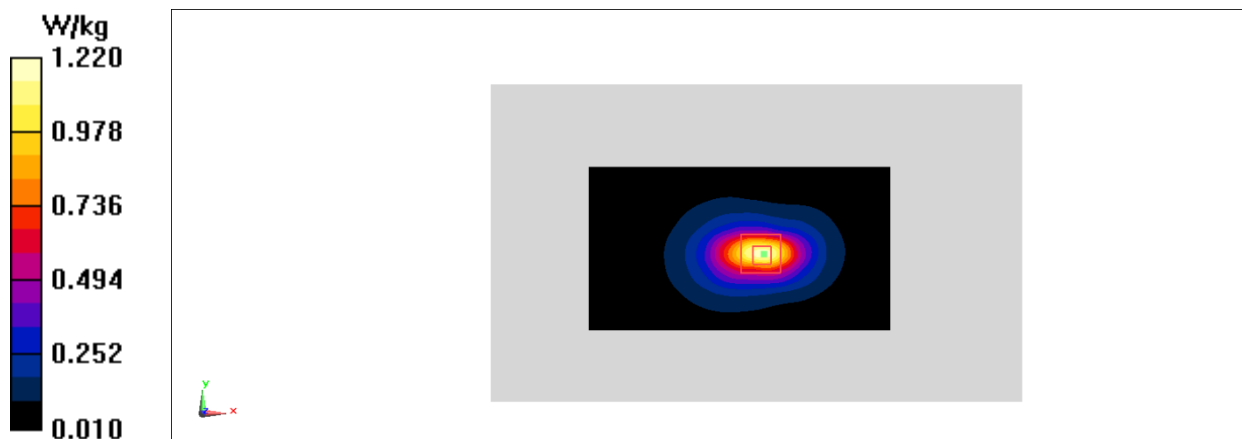
Fig.15 LTE Band2
