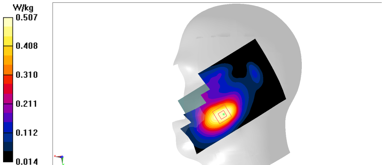
Fig.8 WCDMA1700
