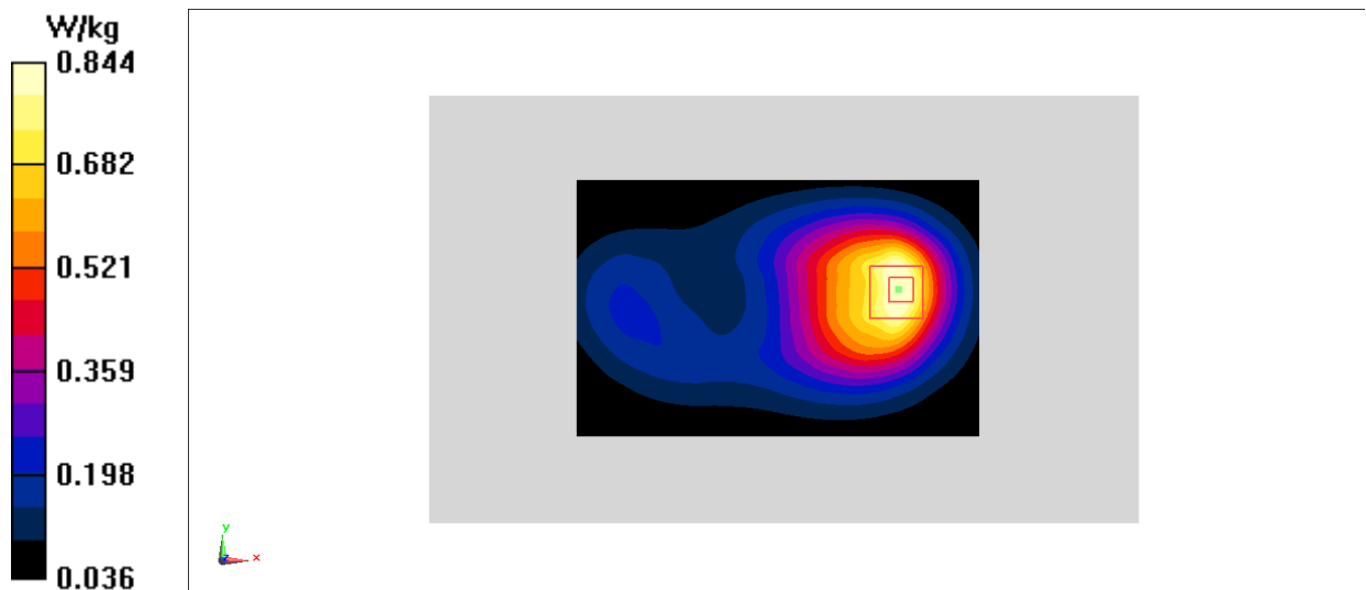
Fig.19 LTE Band4
