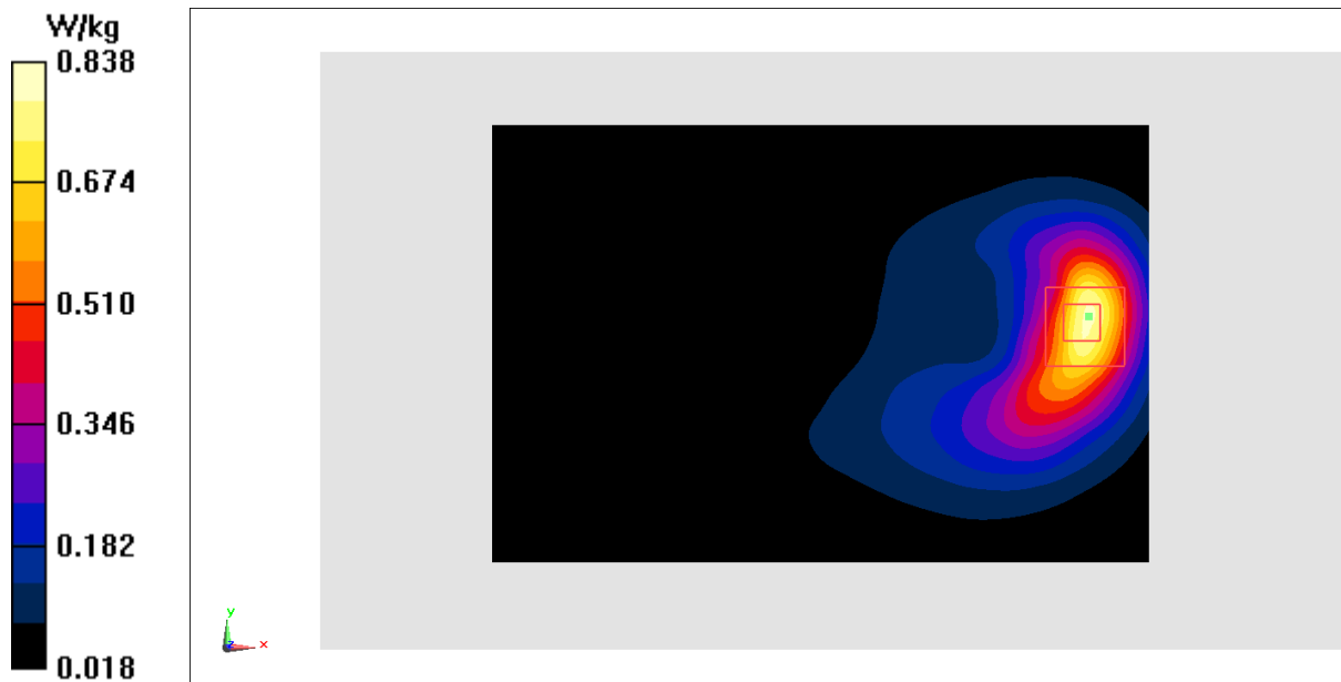
Fig.16 LTE Band2
