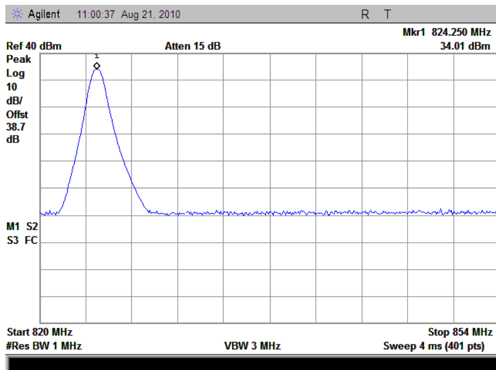
(Plot G: GPRS-TX 850MHz Channel = 128)
