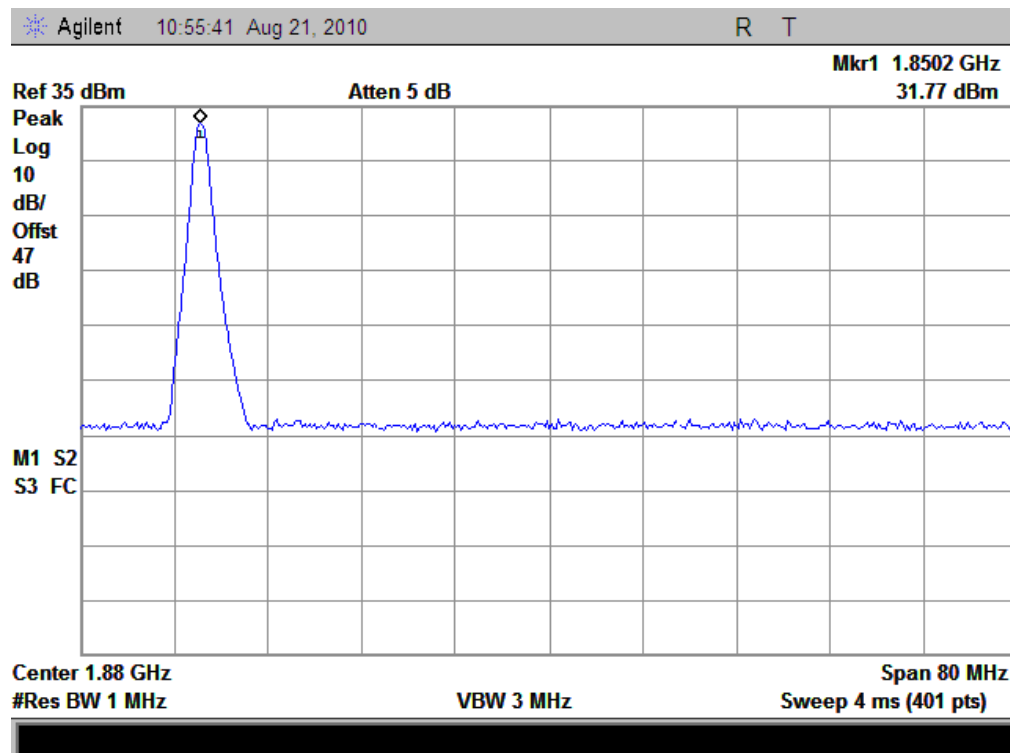
(Plot J: GPRS-TX 1900MHz Channel = 512)
