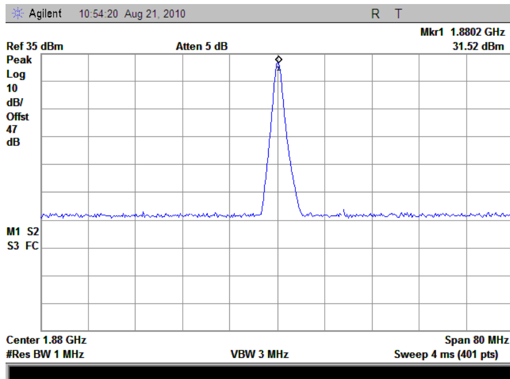
(Plot K: GPRS-TX 1900MHz Channel = 661)
