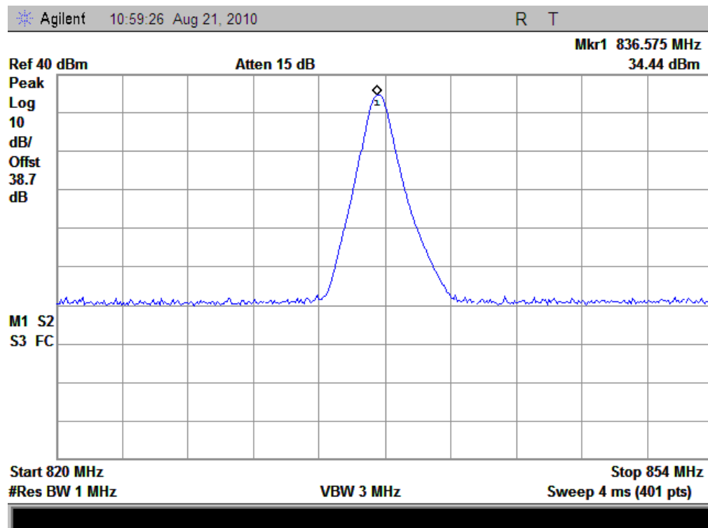
(Plot H: GPRS-TX 850MHz Channel = 190)
