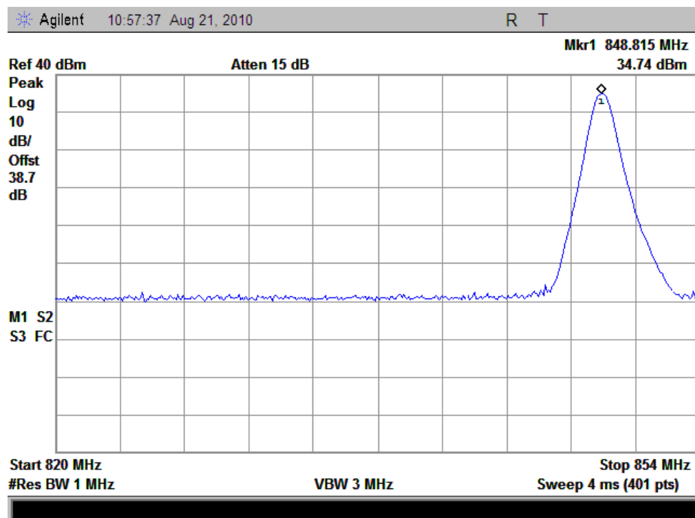
(Plot I: GPRS-TX 850MHz Channel = 251)
