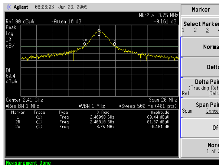
TX Mode 2410MHz
