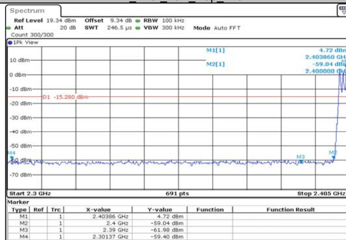
DH1_Ant1_Low_Hop_2402
