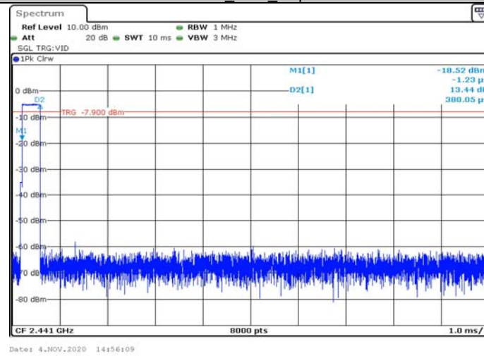
DH1_Ant1_Hop
