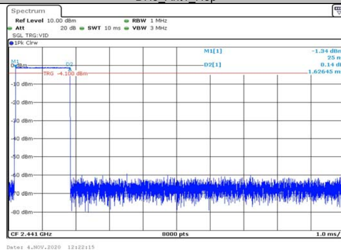
DH3_Ant1_Hop
