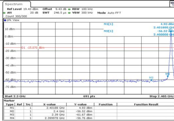
DH1_Ant1_Low_2402
