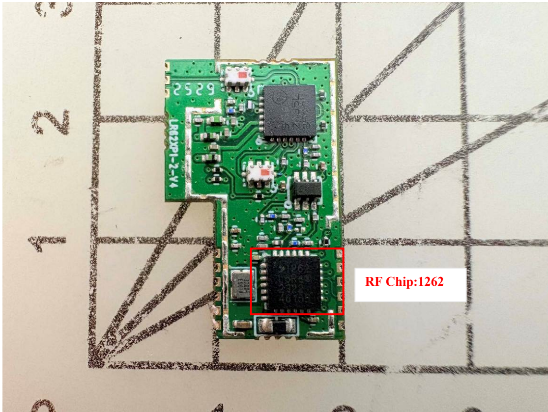
EUT-7. LR62X1P
