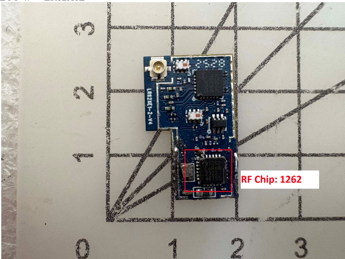
EUT-4. LR62X1E
