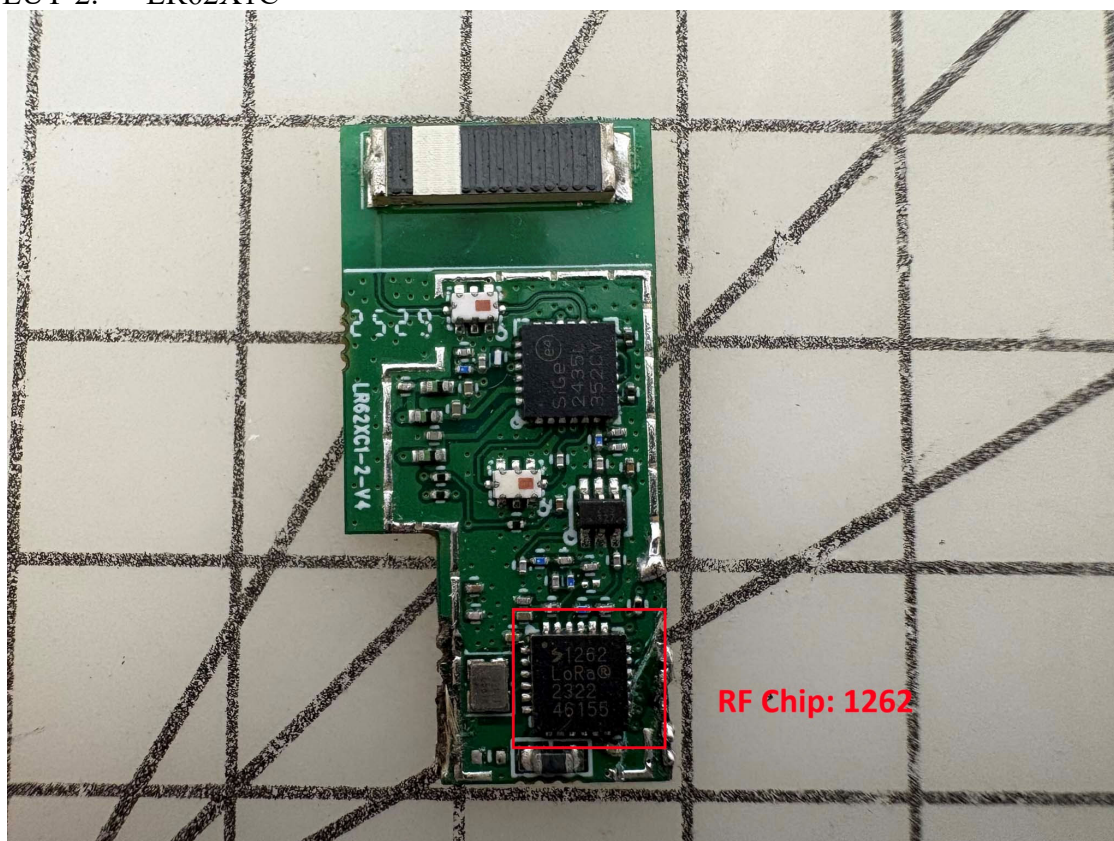
EUT-2. LR62X1C
