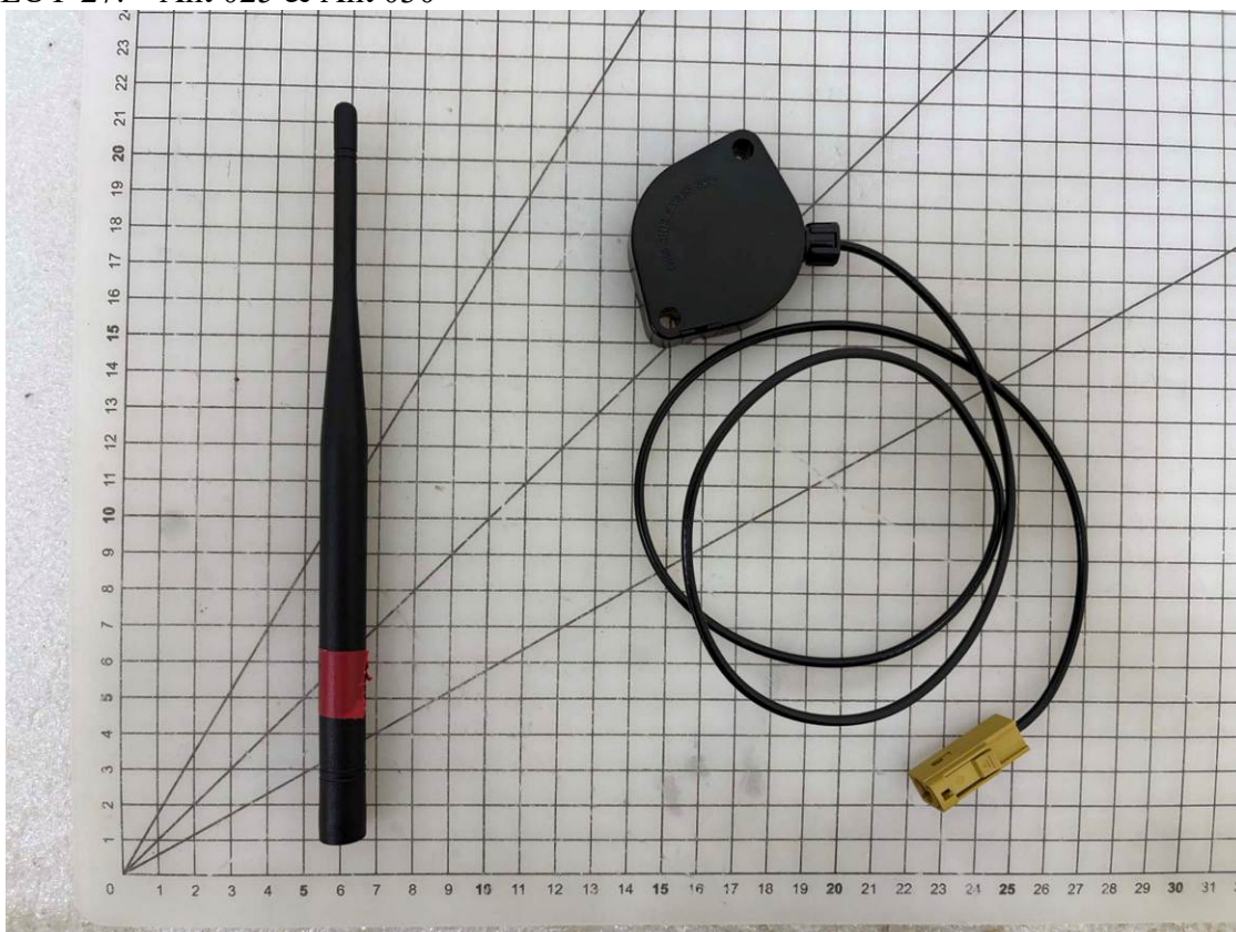
EUT-27. Ant 025 & Ant 030
