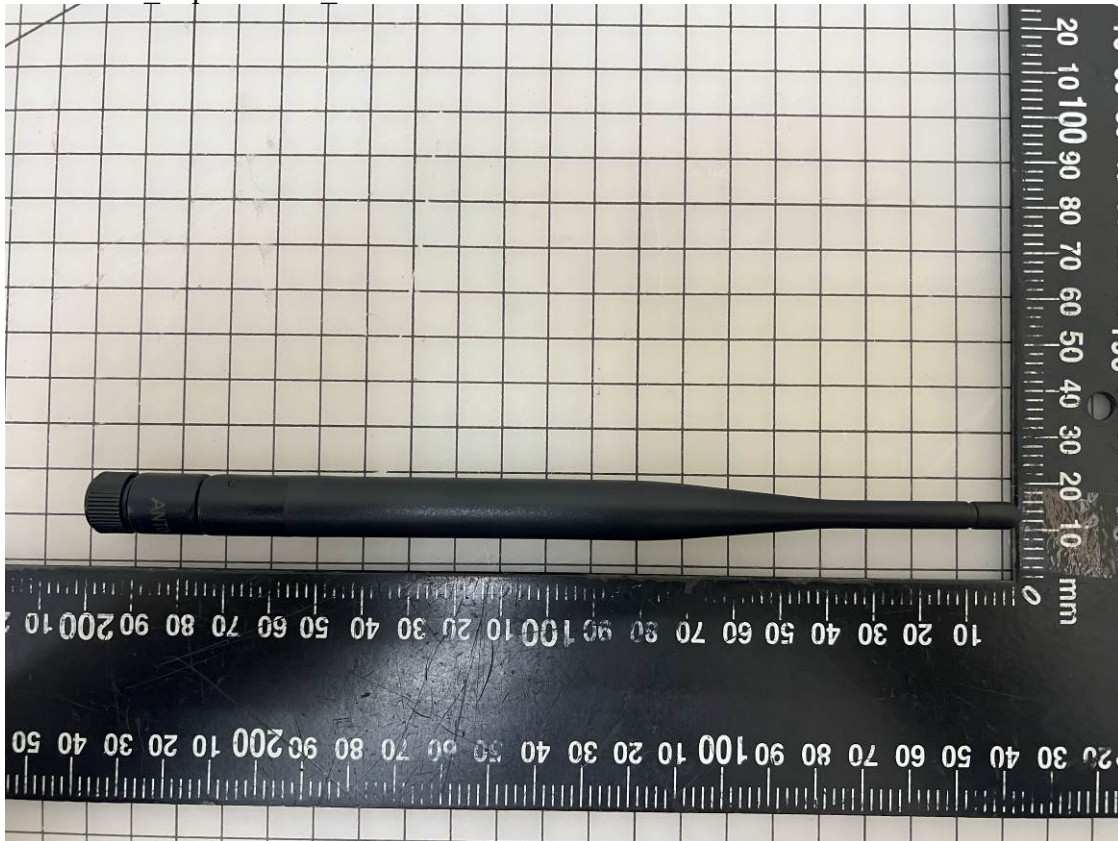
EUT-19. Dipole ANT ANT060
